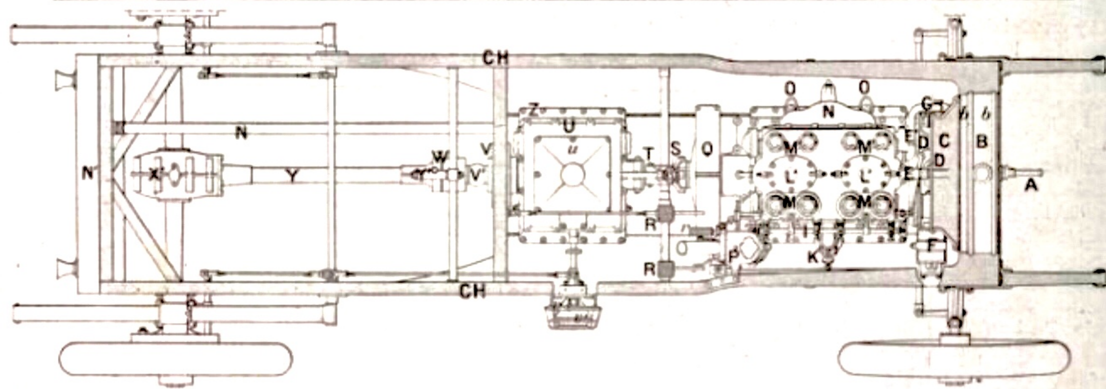
fig. 2. — CHASSIS CORNILIEU ET SAINTE-BEUVE, VU EN ÉLEVATION ET EN PLAN. — A, manivelle de mise en marche. — B, radiateur. — b, /
