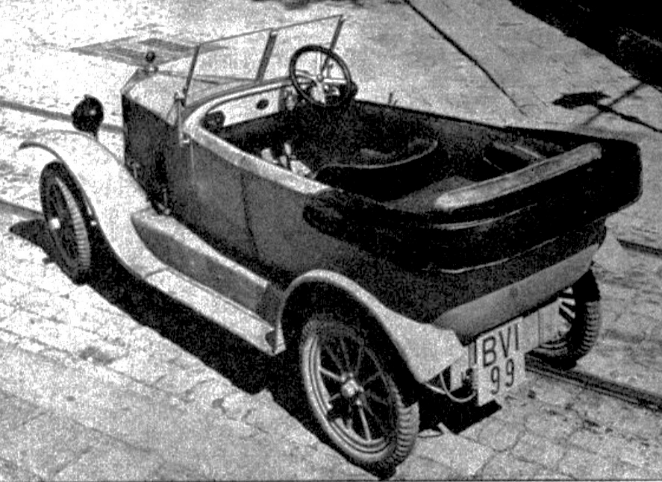
Dreisitziger Fuchs-Wagen, ausgestattet mit 5/15-PS-Fuchs-Serien-Motor der Inzersdorfer Industriewerke.
