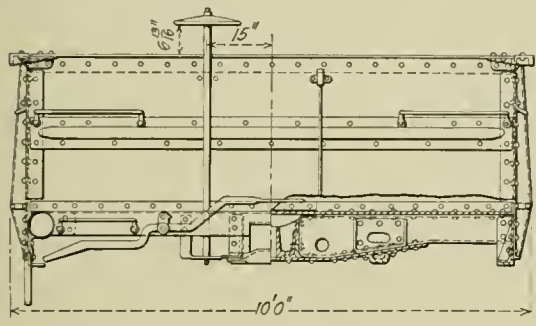
Section A-B.
