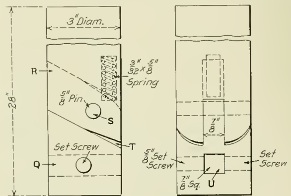
Fig. 3—Slotter Tool Holder
