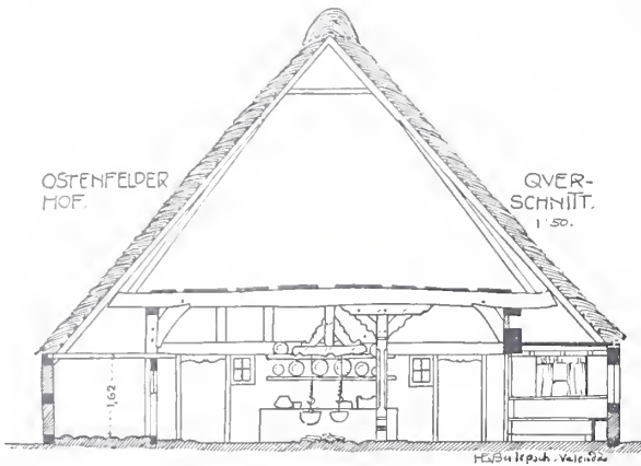
Abb. 36. Bautenmuseum zu Lingby bei Kopenhagen. Querschnitt des Osterfelder Hofes. Aufnahme von Berlepsch-Valendas
