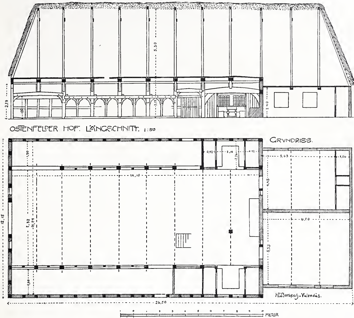
Abb. 35. Bautenmuseum zu Lingby bei Kopenhagen. Grundriß und Längsschnitt des Osterfelder Hofes, Aufnahme von Berlepsch-Valendäs
