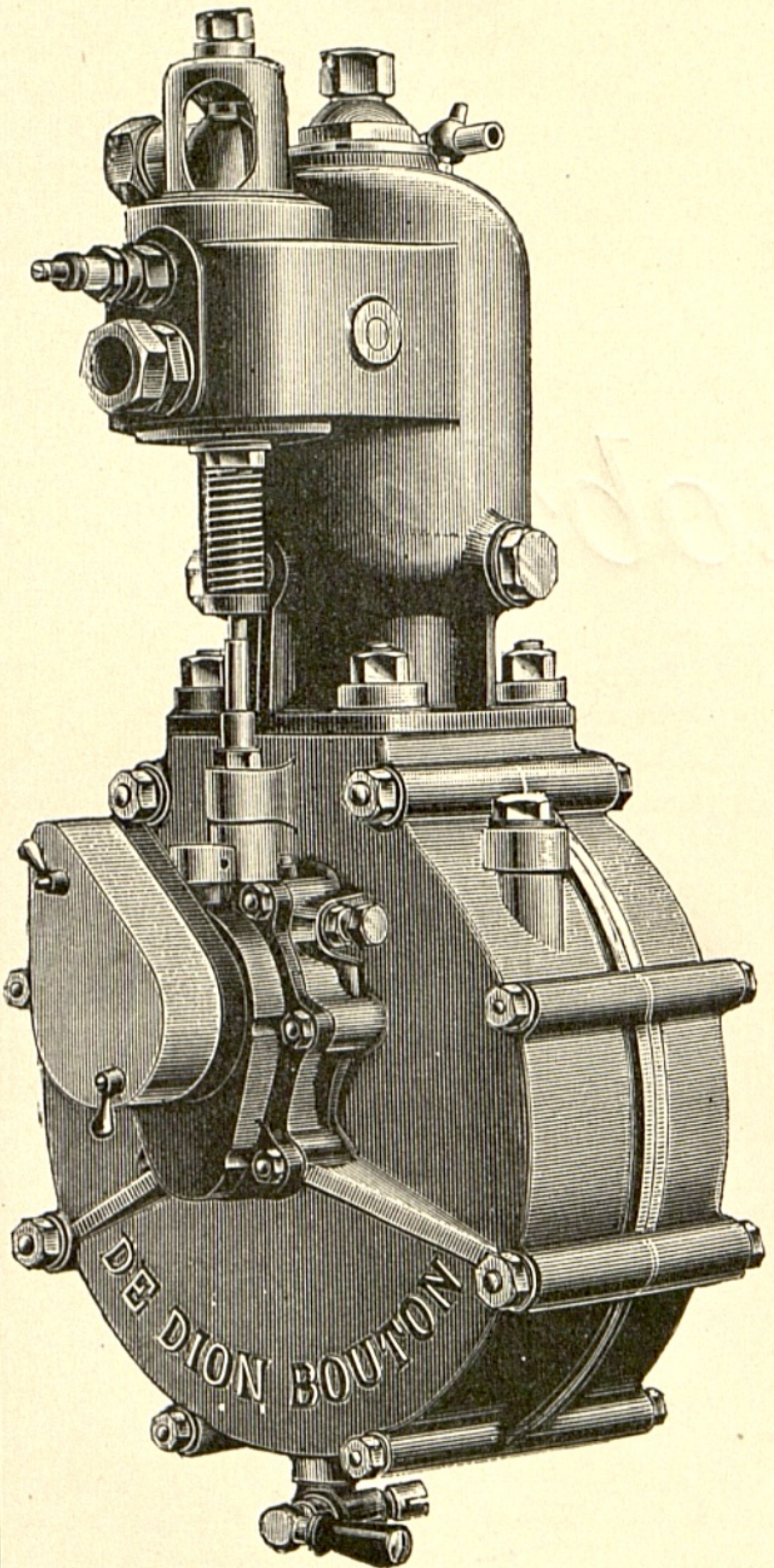
Moteur de la Voiturette
