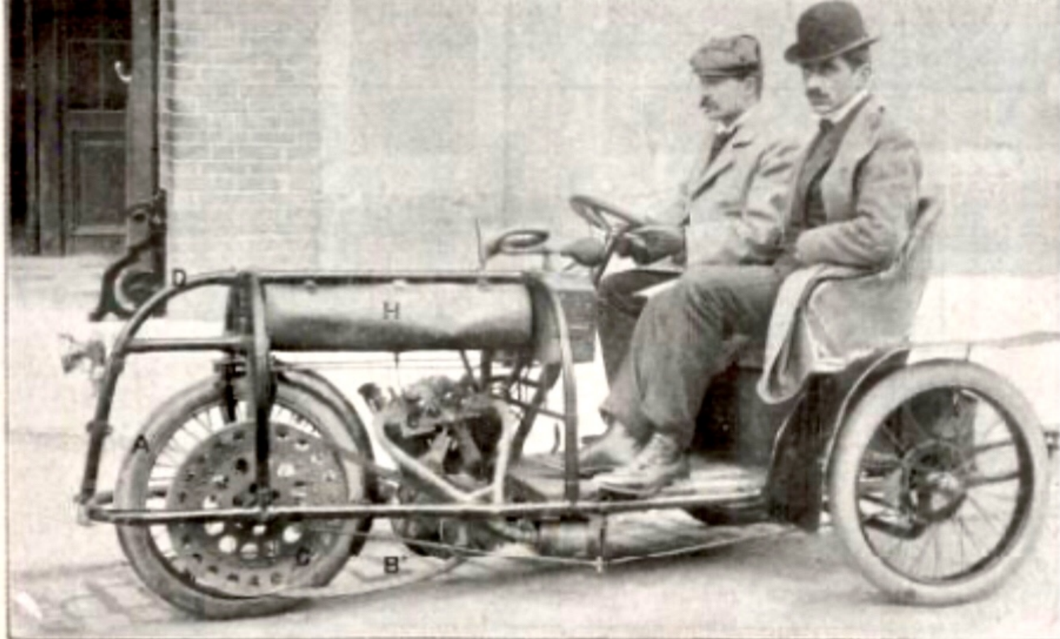
Fig. 2. — TRI-VOITURETTE " ORUS " VUE PAR L'AVANT ET DE CÔTÉ. — A, roue directrice et motrice. — B, joint de cardan. — C, poulie à gorge conique réceptrice. — B', la courroie. — D, bâti en tube. — E, fourche de direction. — F, embrayage. — G, ventilateur du moteur (à 2 cylindres). — H, réservoir à essence et huile.
