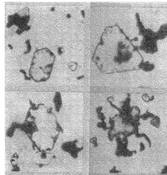
Рис. 6. Отдельные моменты проявления нормально освещенных эмульсионных зерен (лин. увелич. 3300×)
