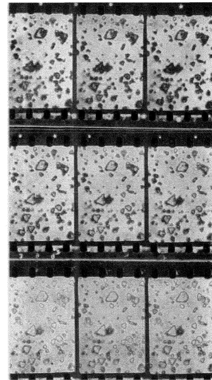
Рис. 9. Киномикрофотография процесса проявления эмульсионных зерен (увеличение с отдельных кадров; лин. увеличен. на кадре 800×)
