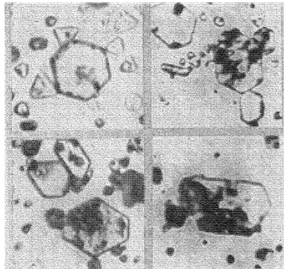
Рис. 4. Микрофотографии эмульсионных зерен, подвергнутых фотохимическому разложению (лин. увелич. 3000×)
