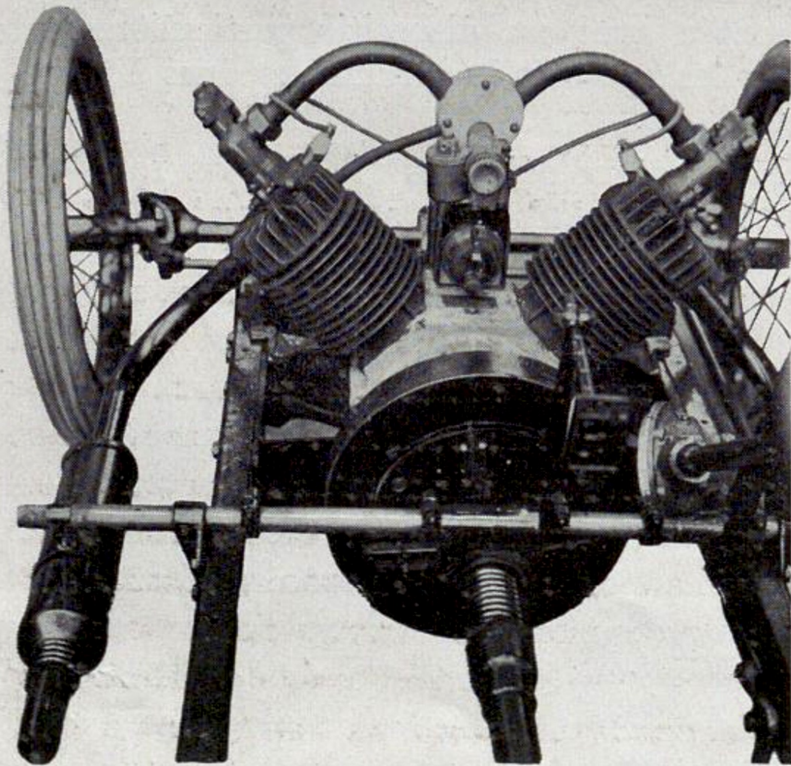
LE MOTEUR DU CYCLECAR G. N. VU PAR L'ARRIÈRE ET L'EMBRAYAGE Entre les deux cylindres, la magnéto et le carburateur.
