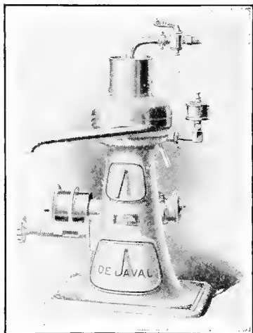
Fig. 23. The DeLaval Centrifugal Emulsifier.
