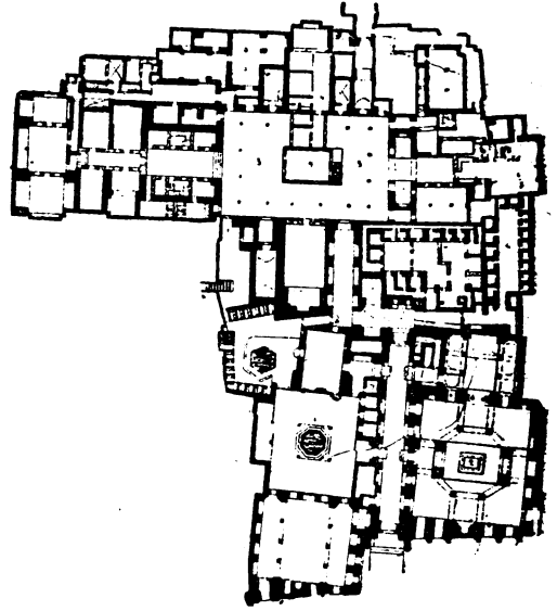
قاهره : مارستانك پلانى
