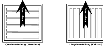
Querbaustellung (Warmbau)
