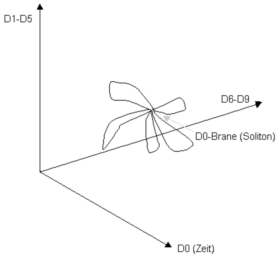
Abbildung 7.3: D0-Brane (=Soliton)
