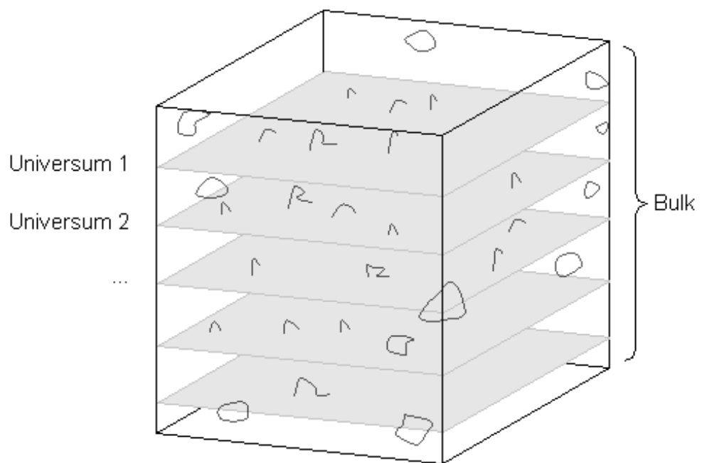
Abbildung 7.5: Bulk
