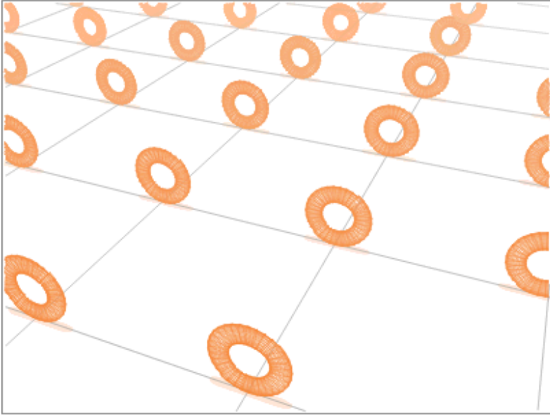
Abb. 13: Zwei Dimensionen zu einem Torus aufgerollt
