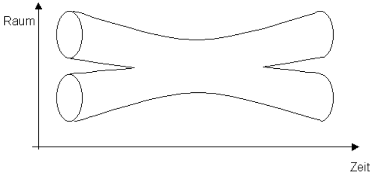
Abb. 8: Vereinigung und anschließende Aufteilung zweier geschlossener Strings
