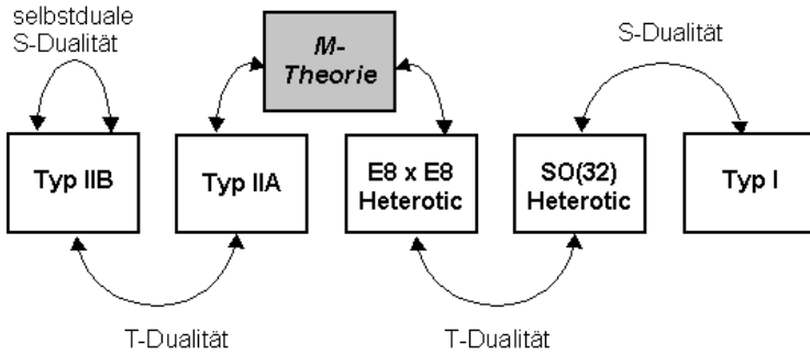
Abb. 23: Dualitäten mit M-Theorie
