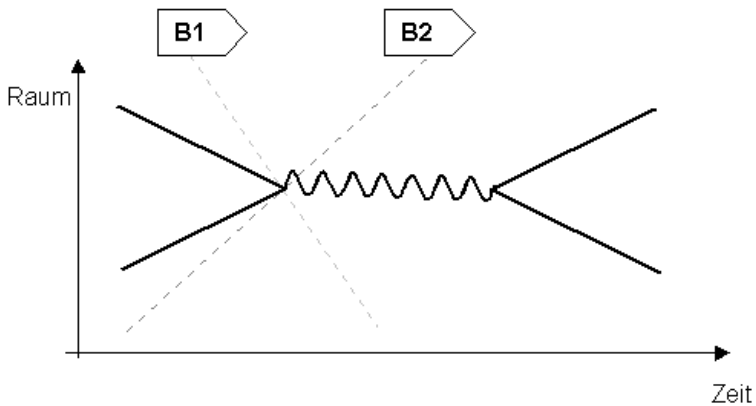
Abb. 9: Feynman Diagramm: Wechselwirkung von Partikeln aus der Sicht zweier sich in Relativbewegung zueinander befindenden Beobachter
