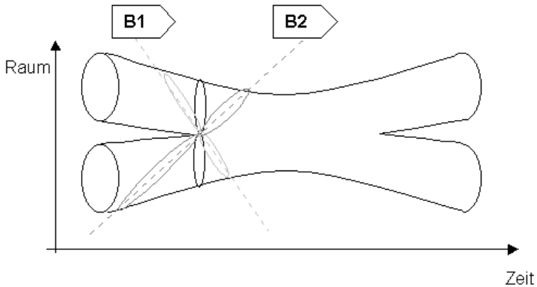
Abb. 10: Wechselwirkung von Strings aus der Sicht zweier sich in Relativbewegung zueinander befindenden Beobachter
