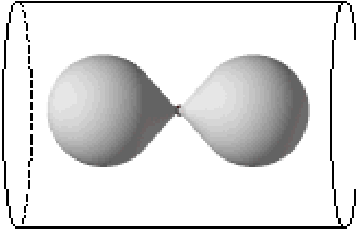
Abb. 18: Weltvolumen eines Strings umhüllt Riss in der Raumzeit
