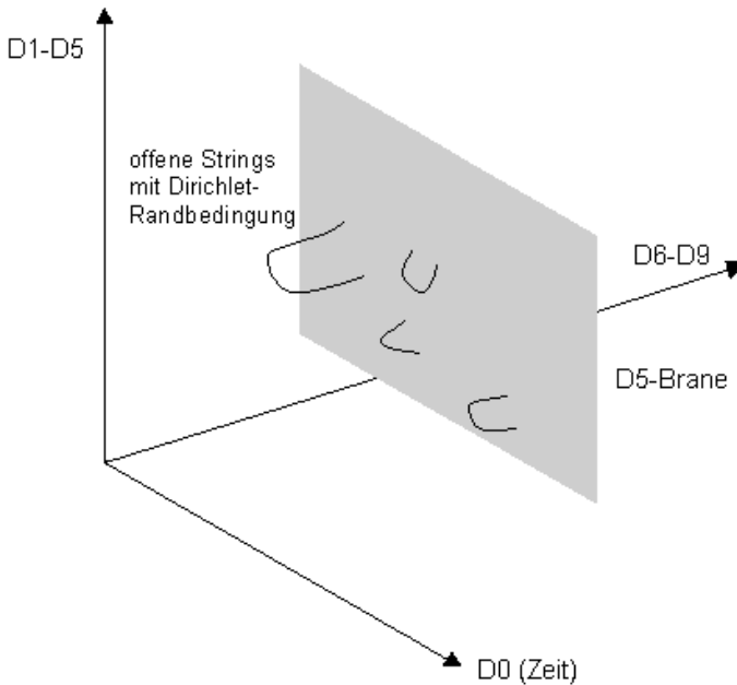
Abb. 25: D-Brane mit Strings, die der Dirichlet-Randbedingung genügen
