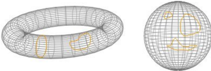
Abb. 14: Strings auf der Oberfläche einer Kugel oder eines Torus
