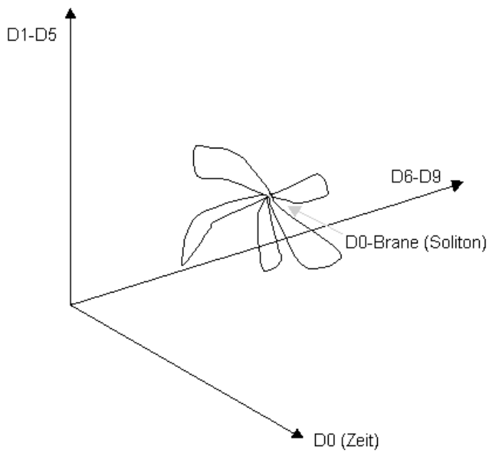
Abb. 27: D0-Bran (=Soliton)
