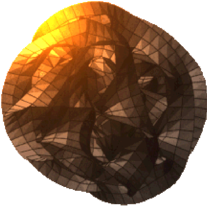
Abb. 15: Calabi-Yau-Mannigfaltigkeit
