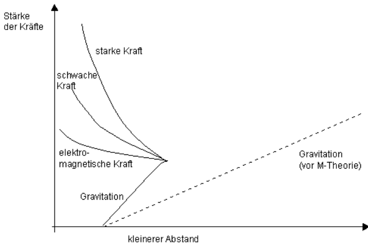
Abb. 24: Vereinigung der Grundkräfte
