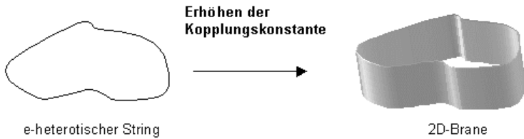
Abb. 21: Erhöhung der Kopplungskonstante beim E-Heterotischen String
