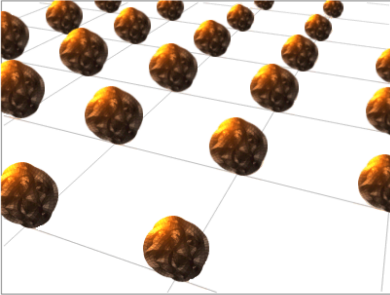
Abb. 16: Calabi-Yau-Mannigfaltigkeiten an jedem Punkt der Raumzeit
