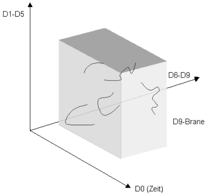
Abb. 26: D9-Bran mit Strings, die der Dirichlet- und der Neumann-Randbedingung genügen
