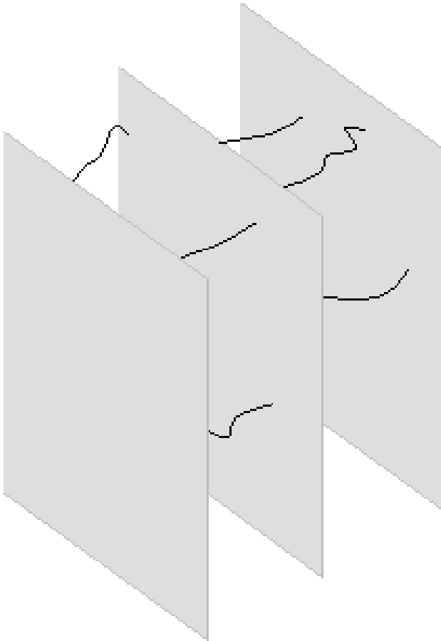
Abb. 28: Strings zwischen D-Branen
