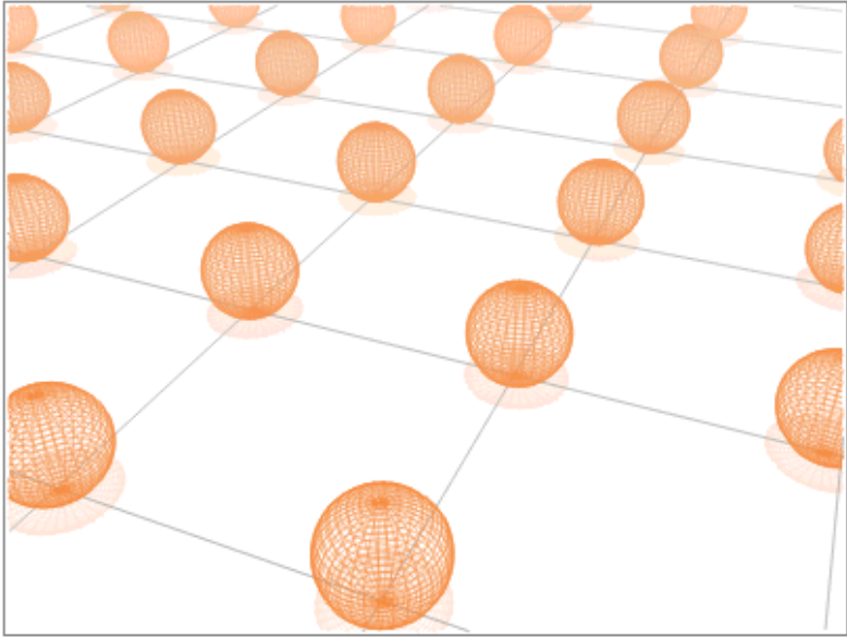
Abb. 12: Zwei Dimensionen zu einer Kugel aufgerollt
