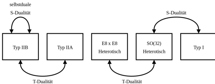
Abb. 20: Dualitäten zwischen den Stringtheorien
