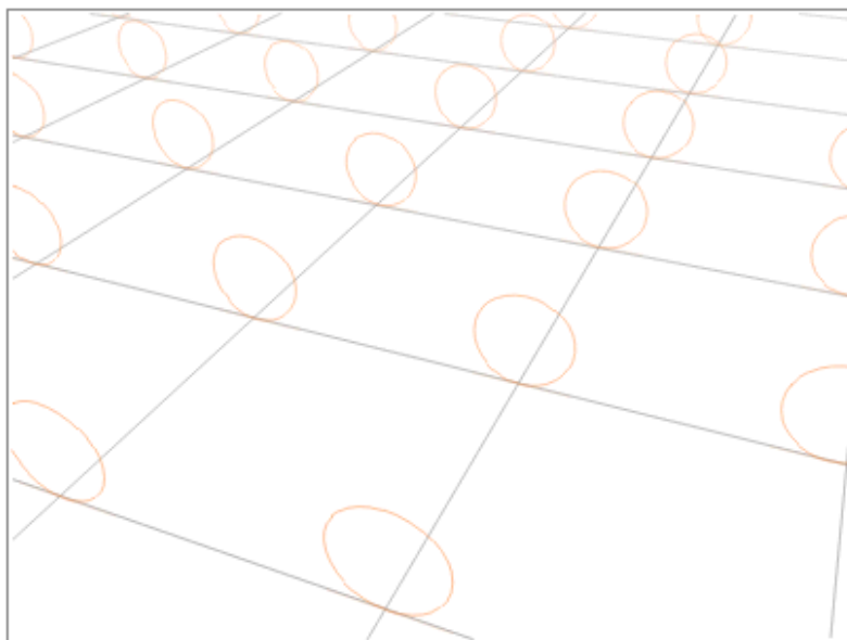
Abb. 11: Eine aufgewickelte Dimension an jedem Punkt der Raumzeit
