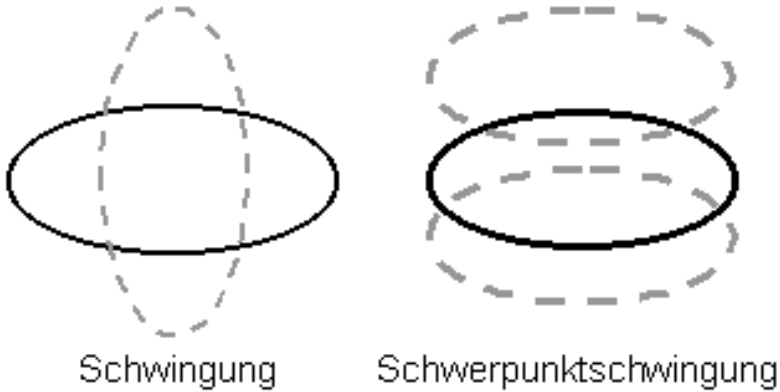
Abb. 5: Schwerpunktschwingung eines Strings
