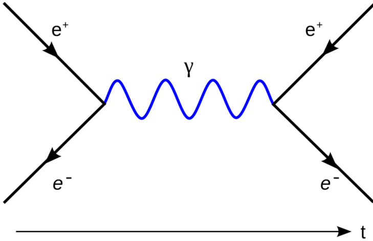
Abb. 6: Punktteilchenwechselwirkung von Elektron und Positron
