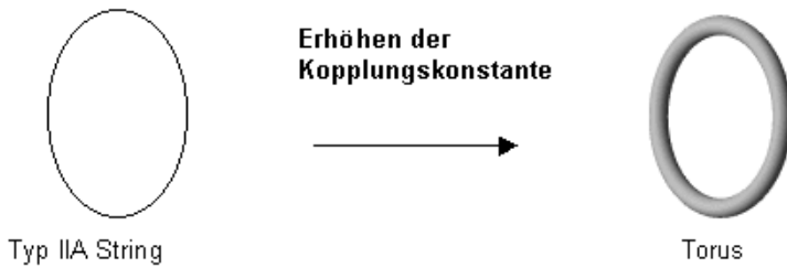
Abb. 22: Erhöhung der Kopplungskonstante beim String vom Typ IIA
