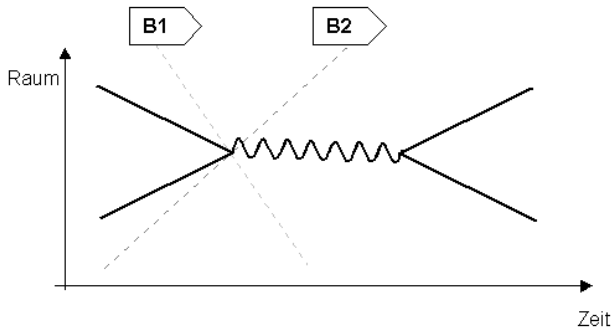
Abb. 7: Feynman Diagramm: Wechselwirkung von Partikeln aus der Sicht zweier sich in Relativbewegung zueinander befindenden Beobachter
