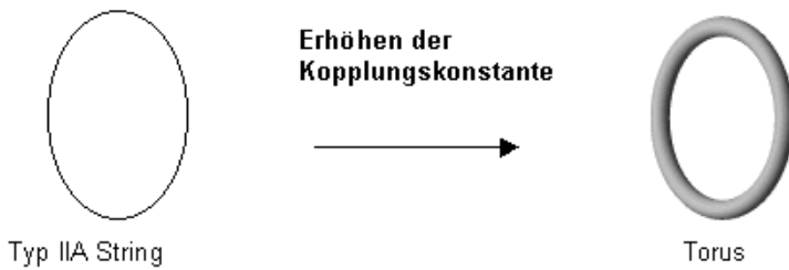
Abb. 20: Erhöhung der Kopplungskonstante beim String vom Typ IIA
