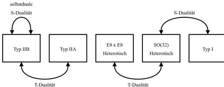
Abb. 18: Dualitäten zwischen den Stringtheorien
