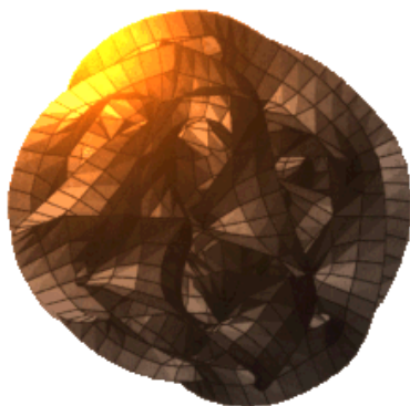
Abb. 13: Calabi-Yau-Mannigfaltigkeit
