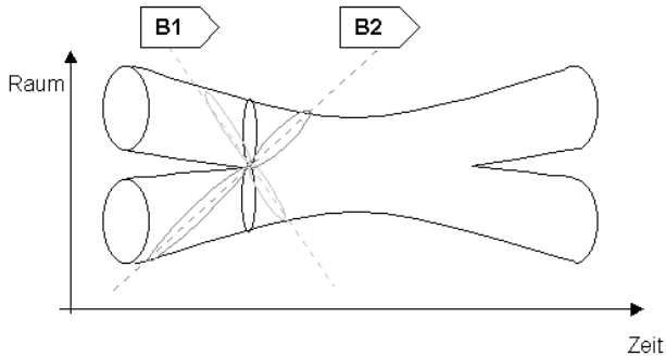
Abb. 8: Wechselwirkung von Strings aus der Sicht zweier sich in Relativbewegung zueinander befindenden Beobachter
