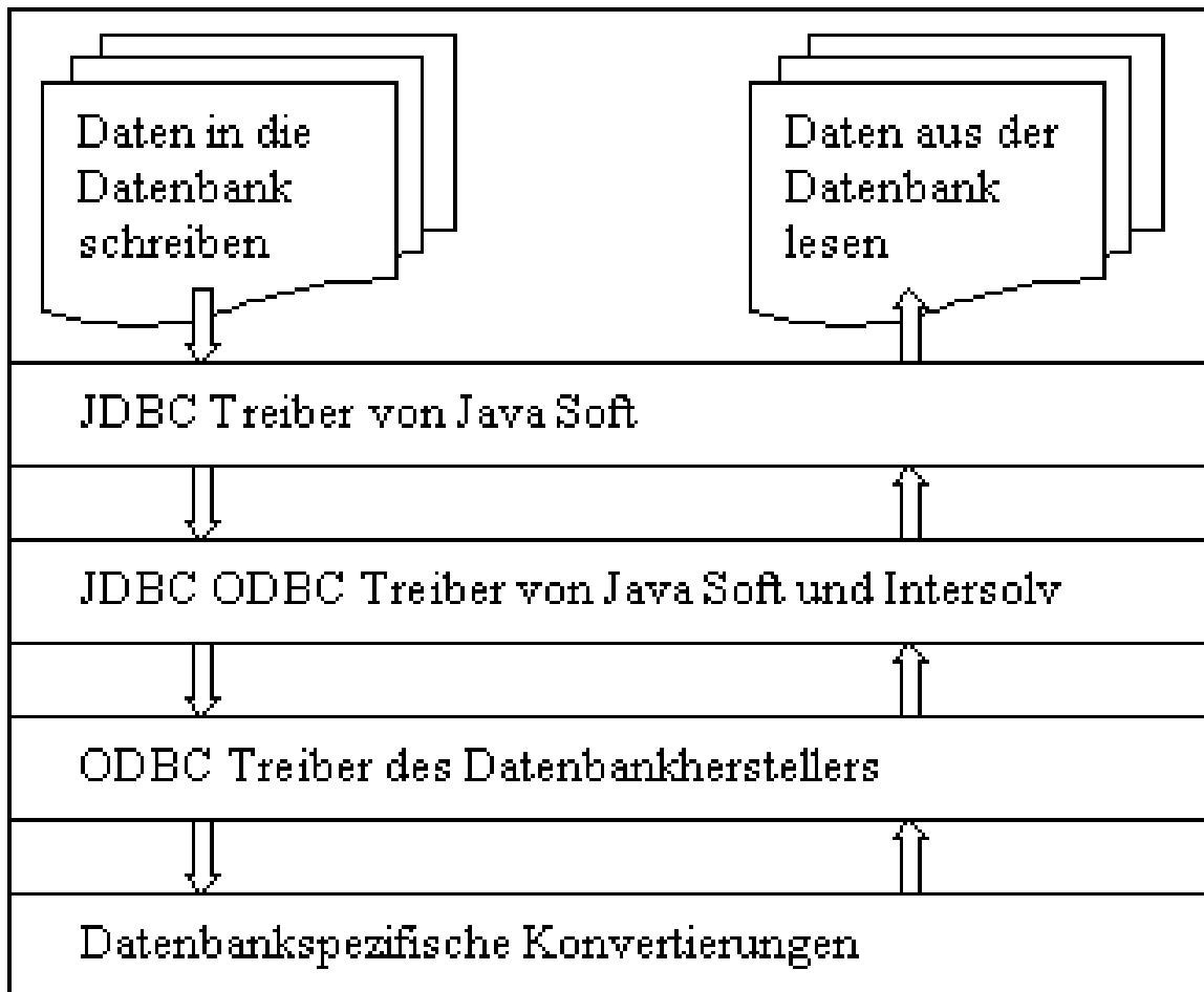
Abb. 9 Konvertierungen bei Datenbankzugriff über die JDBC ODBC Brücke
