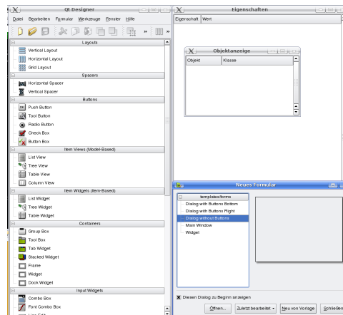
Abbildung 10: Unser Dialogfenster
