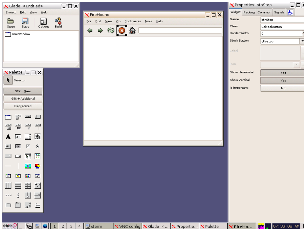
Abbildung 13: Das Hauptfenster
