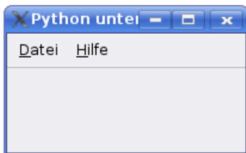
Abbildung 7: guiqt3.py Anwendung
