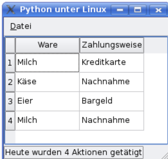
Abb. 8 guiqt3.py Anwendung
