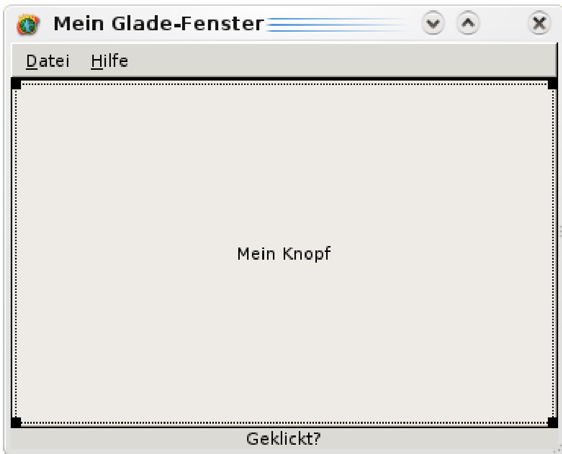
Abb. 15 Das Hauptfenster
