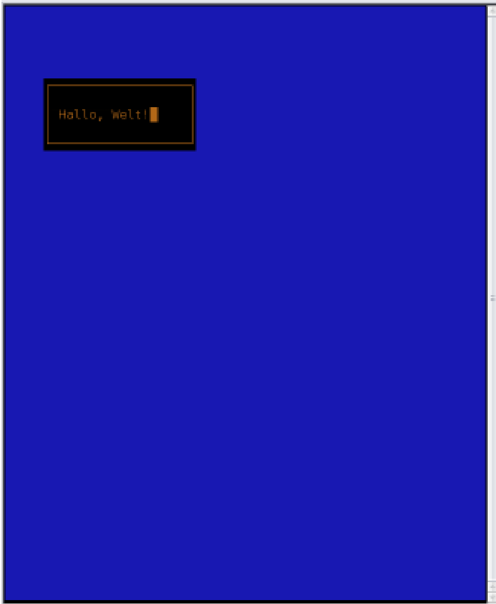
Abb. 17 Hallo Welt
