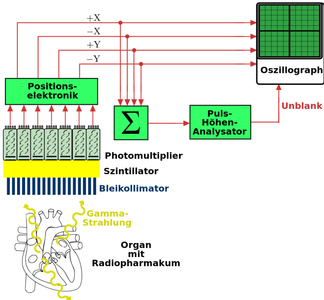
Abb. 52 Blockdiagramm einer Gammakamera
