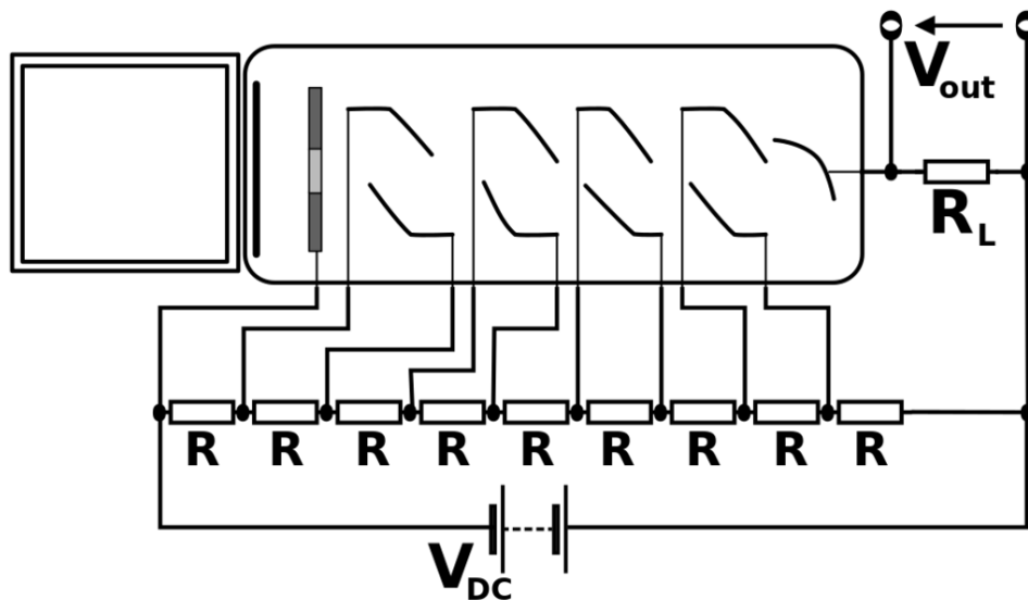
Abb. 39 Schemazeichnung einer Photomultiplerröhre mit Beschaltung
