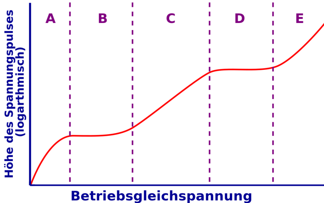
Abb. 29 Betriebsarten eines gasgefüllten Strahlungsdetektors
