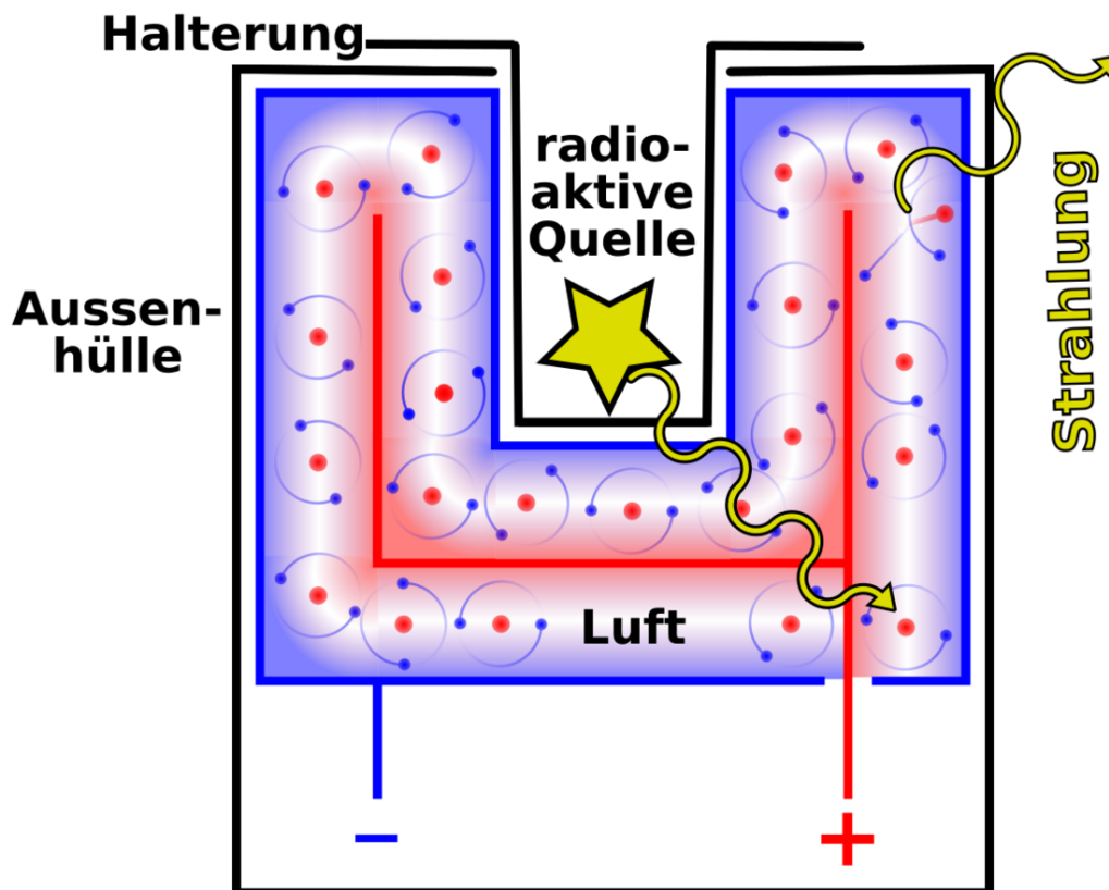
Abb. 30 Dosiskalibrator (schematisch)
