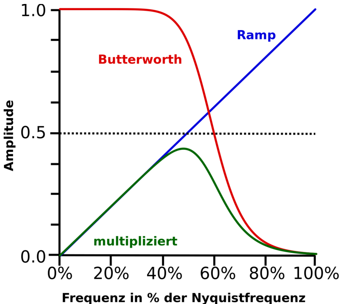
Abb. 152 Ramp- und Butterworthfilter (Fünfte Ordnung 60% Cutoff)
