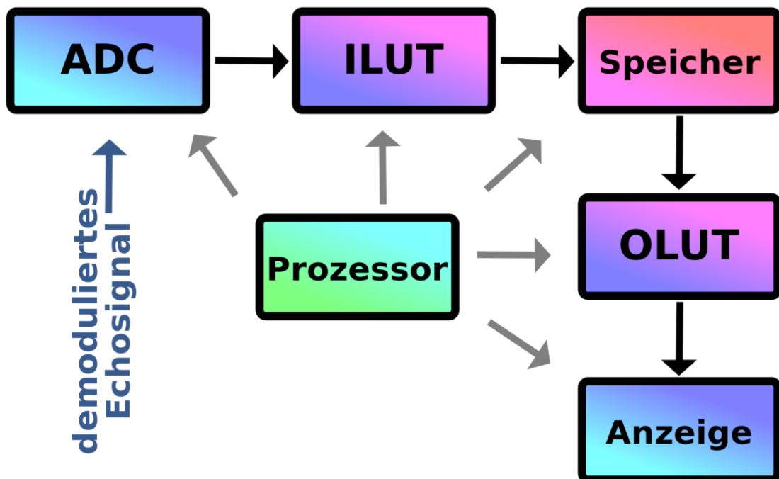
Abb. 168 Vereinfachtes Blockdiagramm der Elektronik eines B-Mode Ultraschallgerätes.
