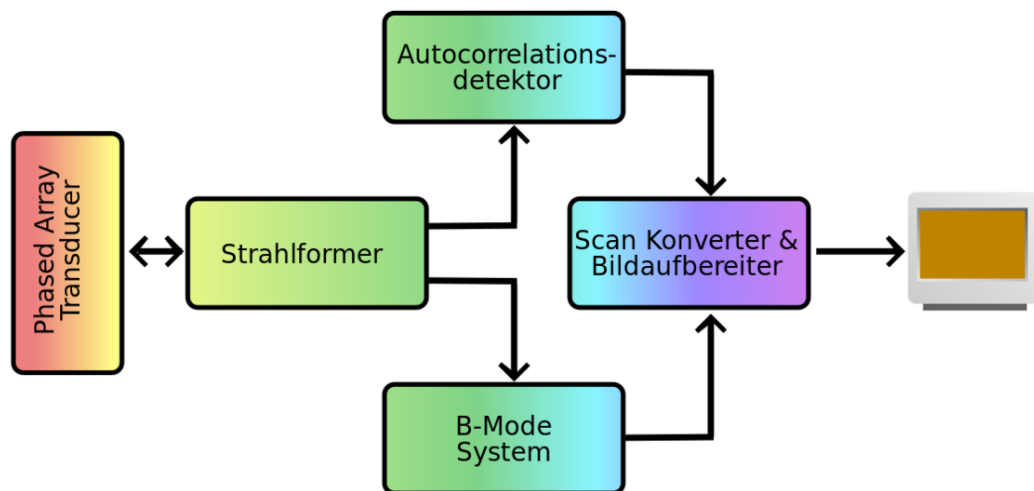
Abb. 178 Blockdiagramm eines System zur Erstellung Flussgeschwindigkeitscodierter Dopplersonogramme
