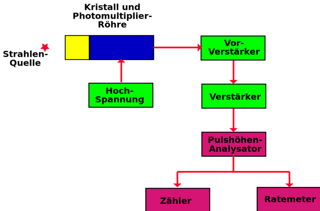
Abb. 50 Einfaches Szintillationsspektrometer
