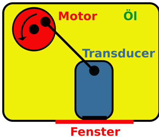
Abb. 166 Mechanischer Transducer als Kolbenmaschine
