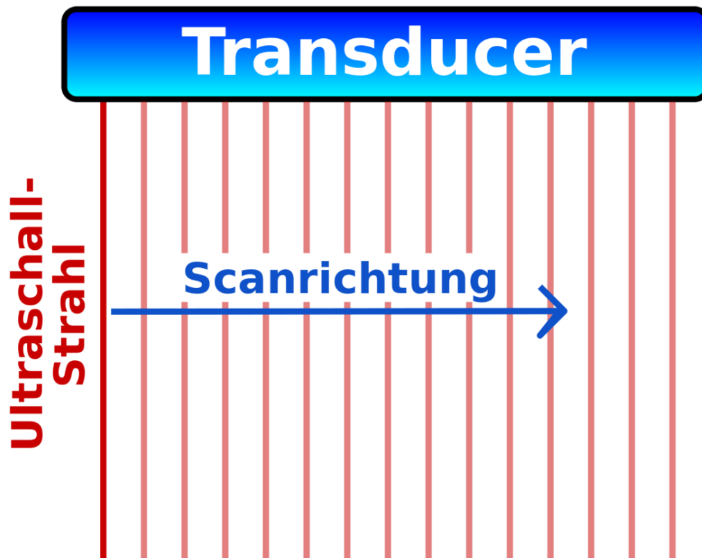
Abb. 163 Vereinfachtes Blockdiagramm eines Ultraschallscanners, mit linearer Transducer Anordnung
