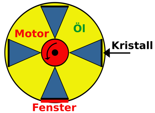
Abb. 167 Mechanischer Transducer mit rotierenden Kristallen
