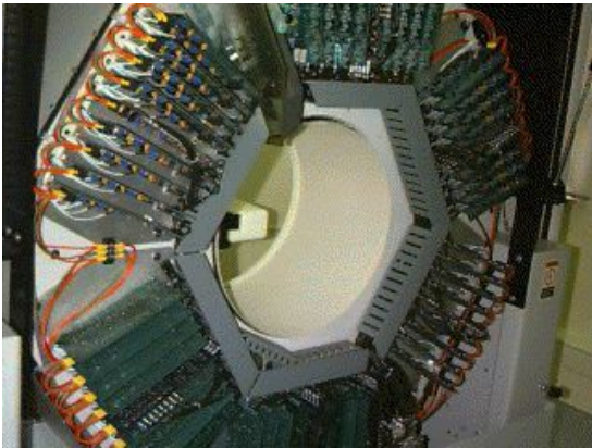
Abb. 90 Die Detektoren mit zugehöriger Elektronik.
