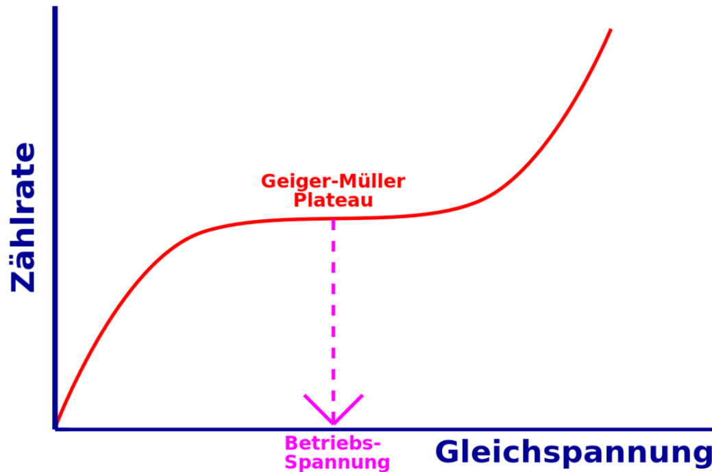
Abb. 37 Betriebsspannung eines Geigerzählers
