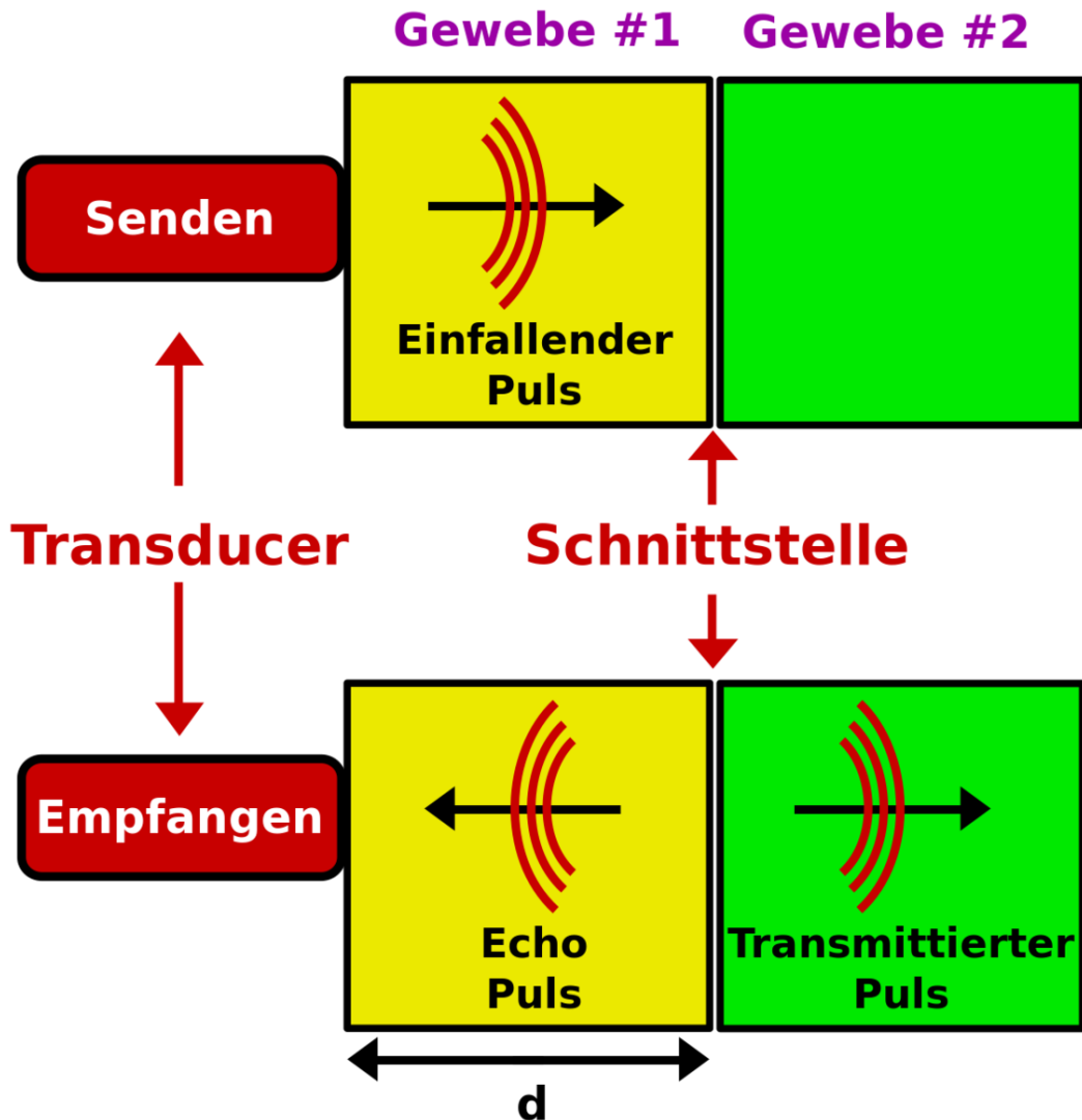
Abb. 160 Darstellung des Puls Echo Prinzips bei der Ultraschall-Bildgebung
