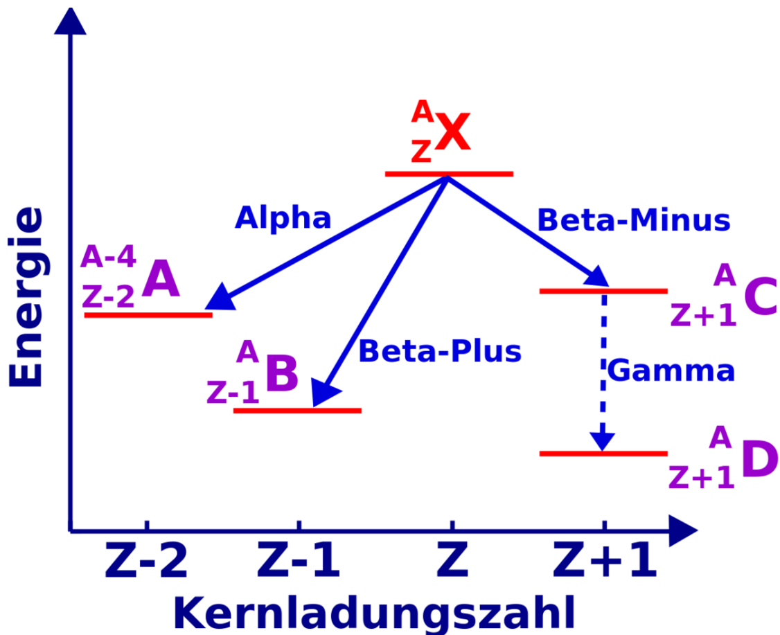
Abb. 7 Allgemeines Zerfallsschema
