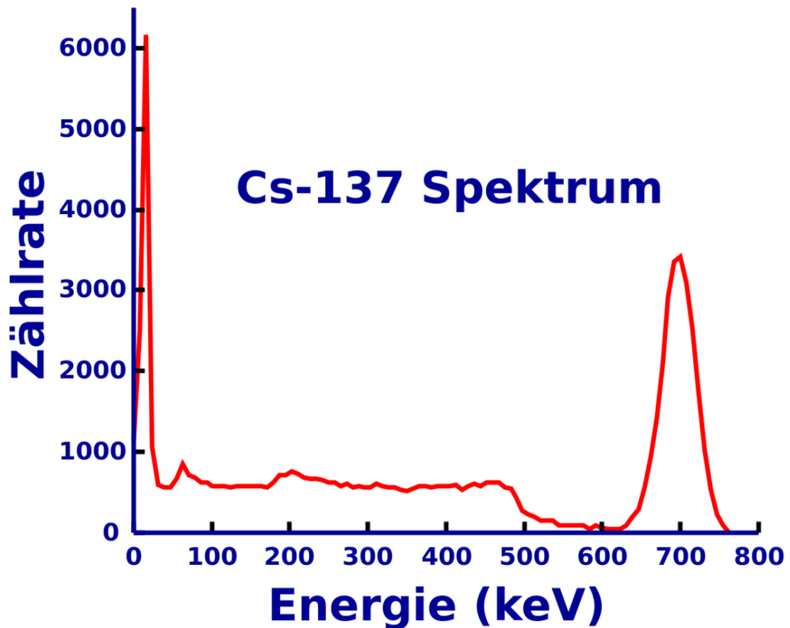
Abb. 48 Gammaskpektrum von Caesium-137
