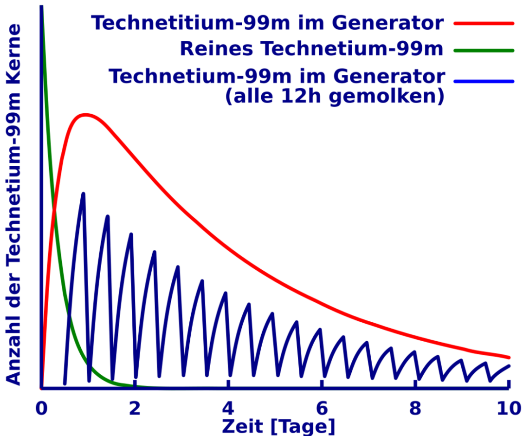
Abb. 98 Zeitlicher Verlauf der Aktivität im Technetium-99m Generator
