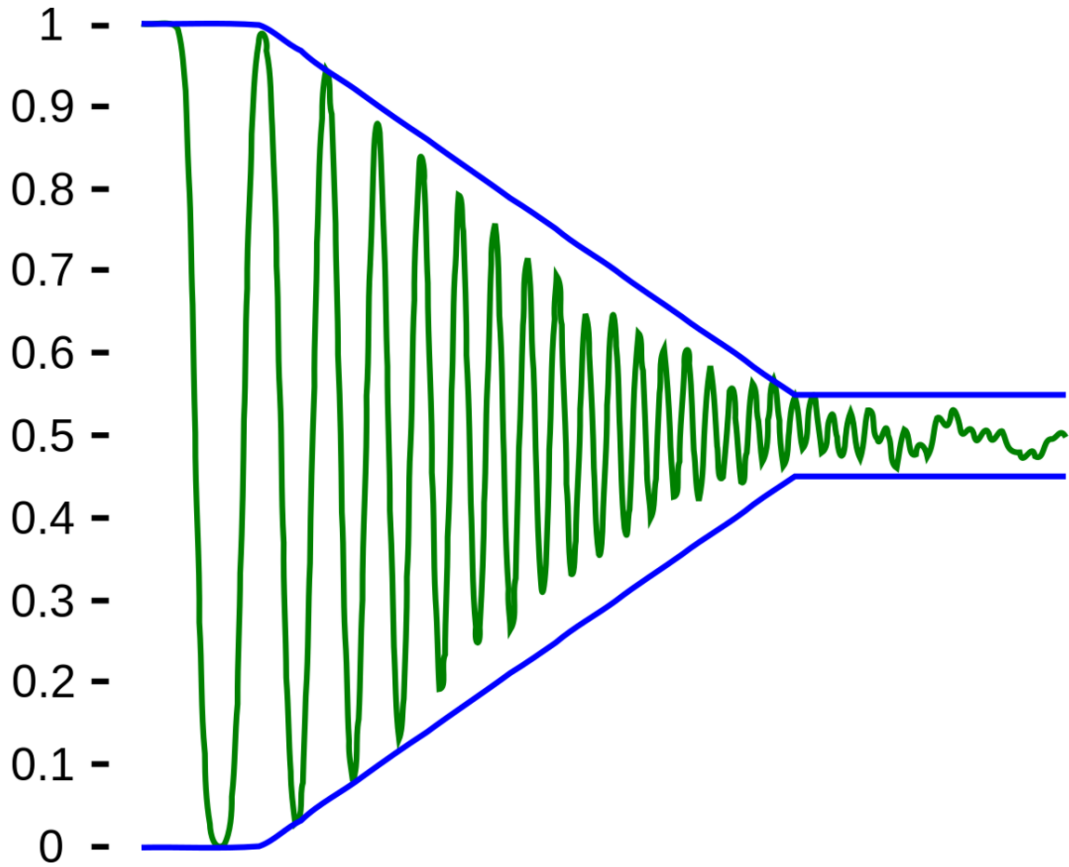
Abb. 138 reales abbildendes System mit blauer Einhüllender
