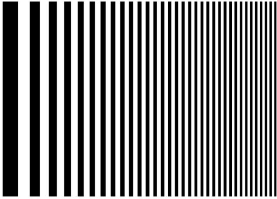
Abb. 135 (Nahezu) ideales abbildendes System
