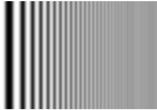
Abb. 136 reales abbildendes System
