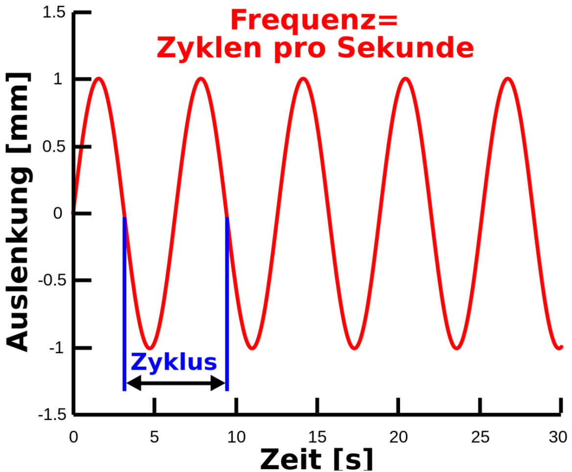
Abb. 131 zeitlicher Verlauf einer Sinuswelle
