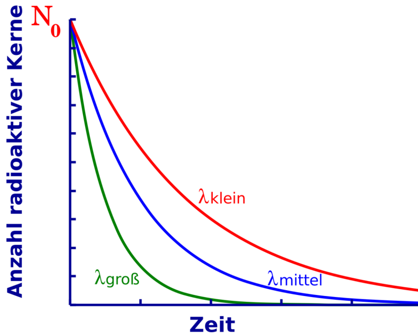
Abb. 9 Exponentieller Zerfall von Kernen in Abhängigkeit von der Zerfallskonstante
