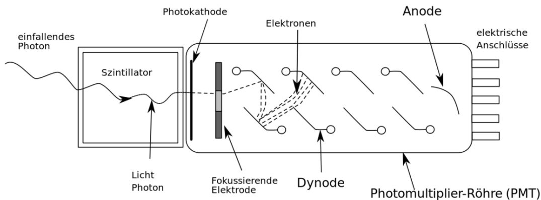
Abb. 38 Schemazeichnung einer Photomultiplierröhre
