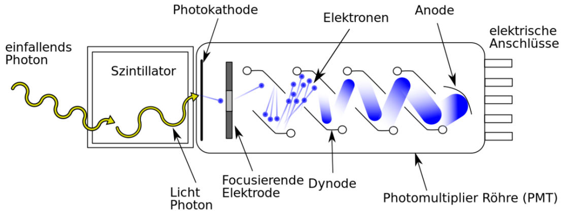
Abb. 40 Schemazeichnung einer Photomultiplierröhre im Betrieb
