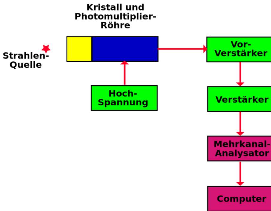
Abb. 51 Komplexes Szintillationsspektrometer
