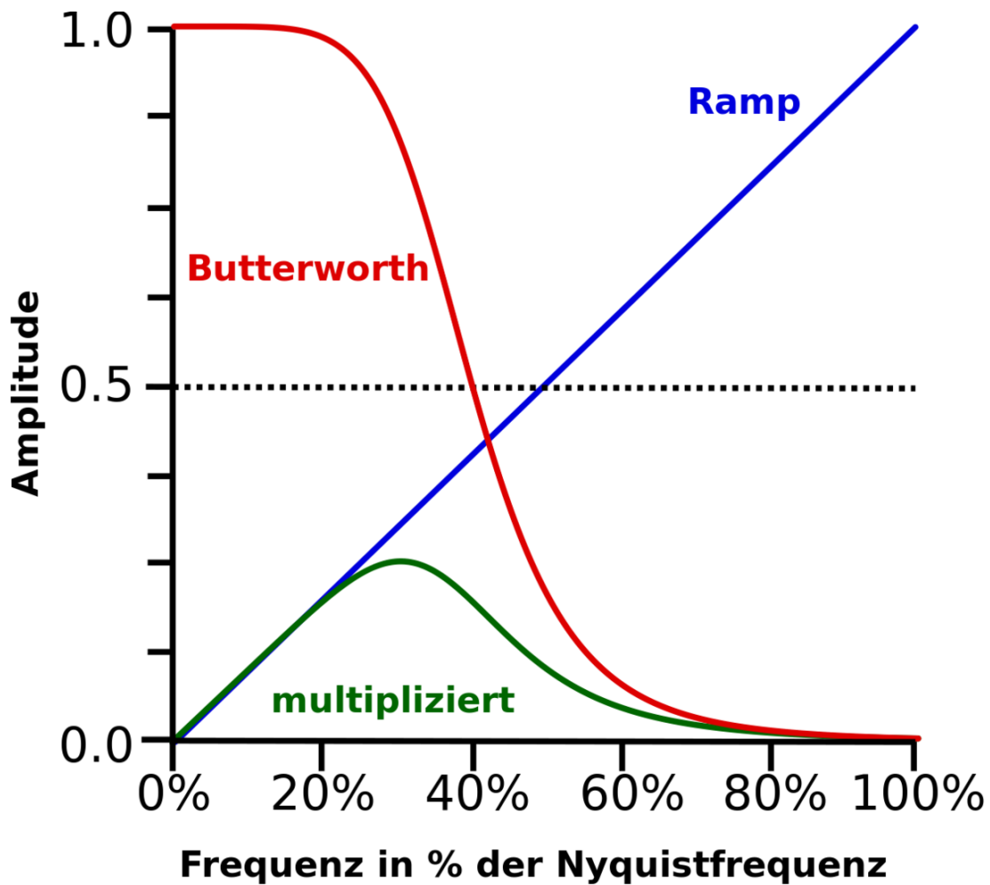
Abb. 154 Ramp- und Butterworthfilter (Dritte Ordnung 40% Cutoff)
