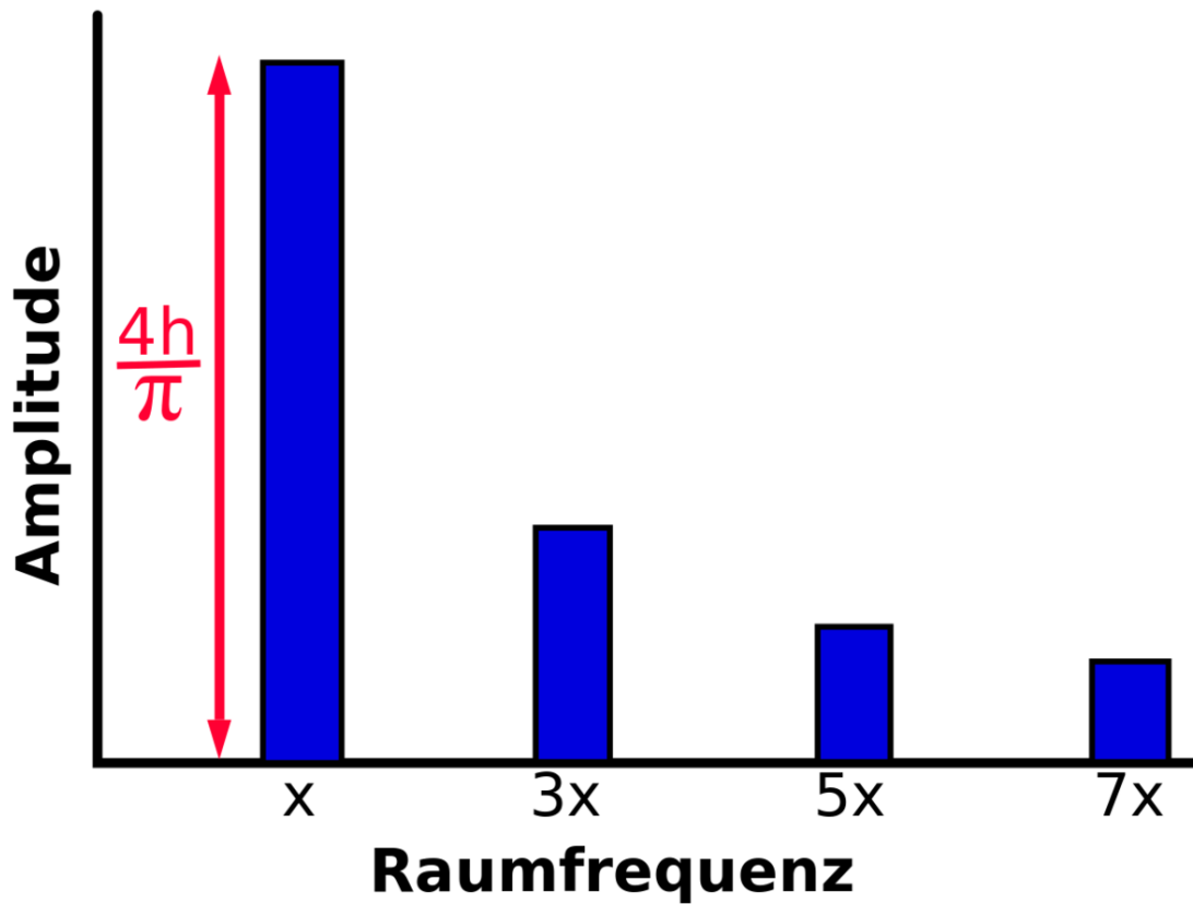
Abb. 145 Fourierspektrum einer Rechteckwelle.
