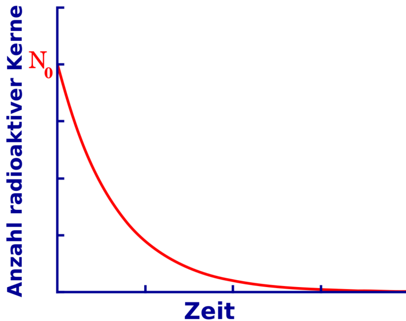
Abb. 8 Exponentieller Zerfall von Kernen
