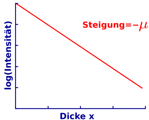
Abb. 24 Exponentielle Dämpfung von Strahlung in logarithmischer Darstellung
