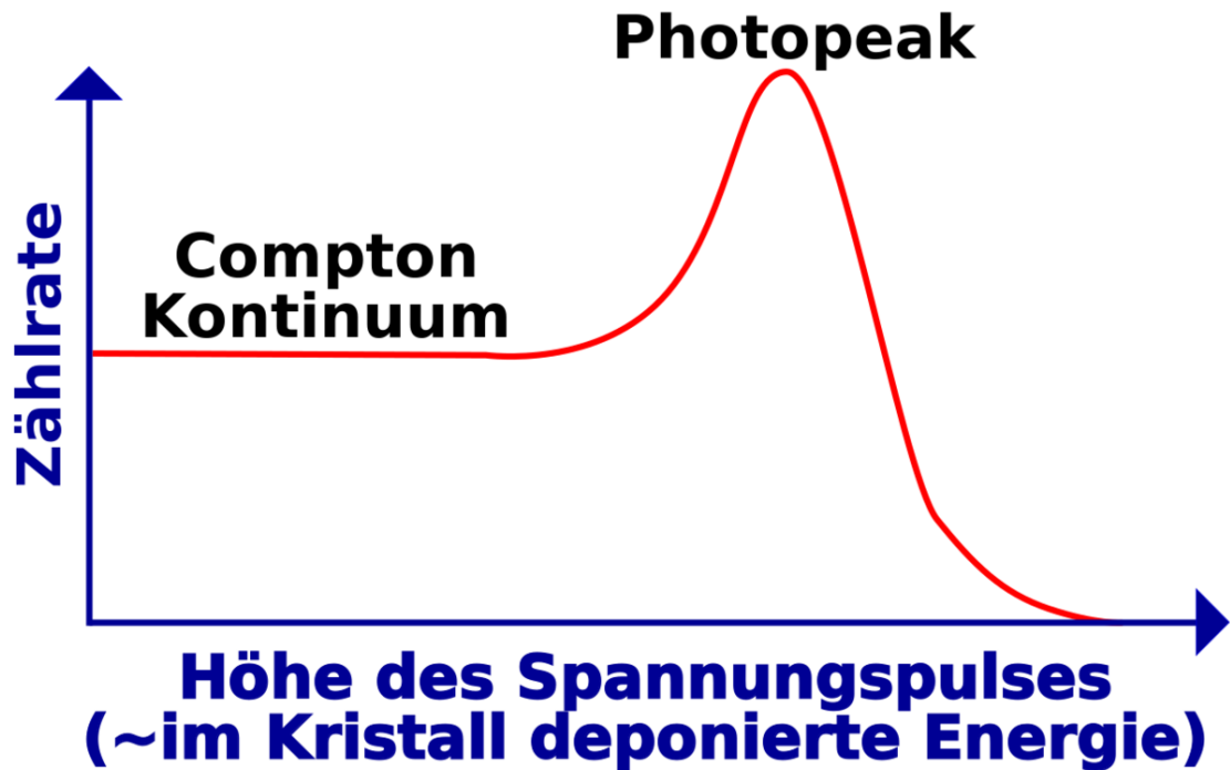
Abb. 47 Gammaspektrum eines monoenergetischen Strahlers
