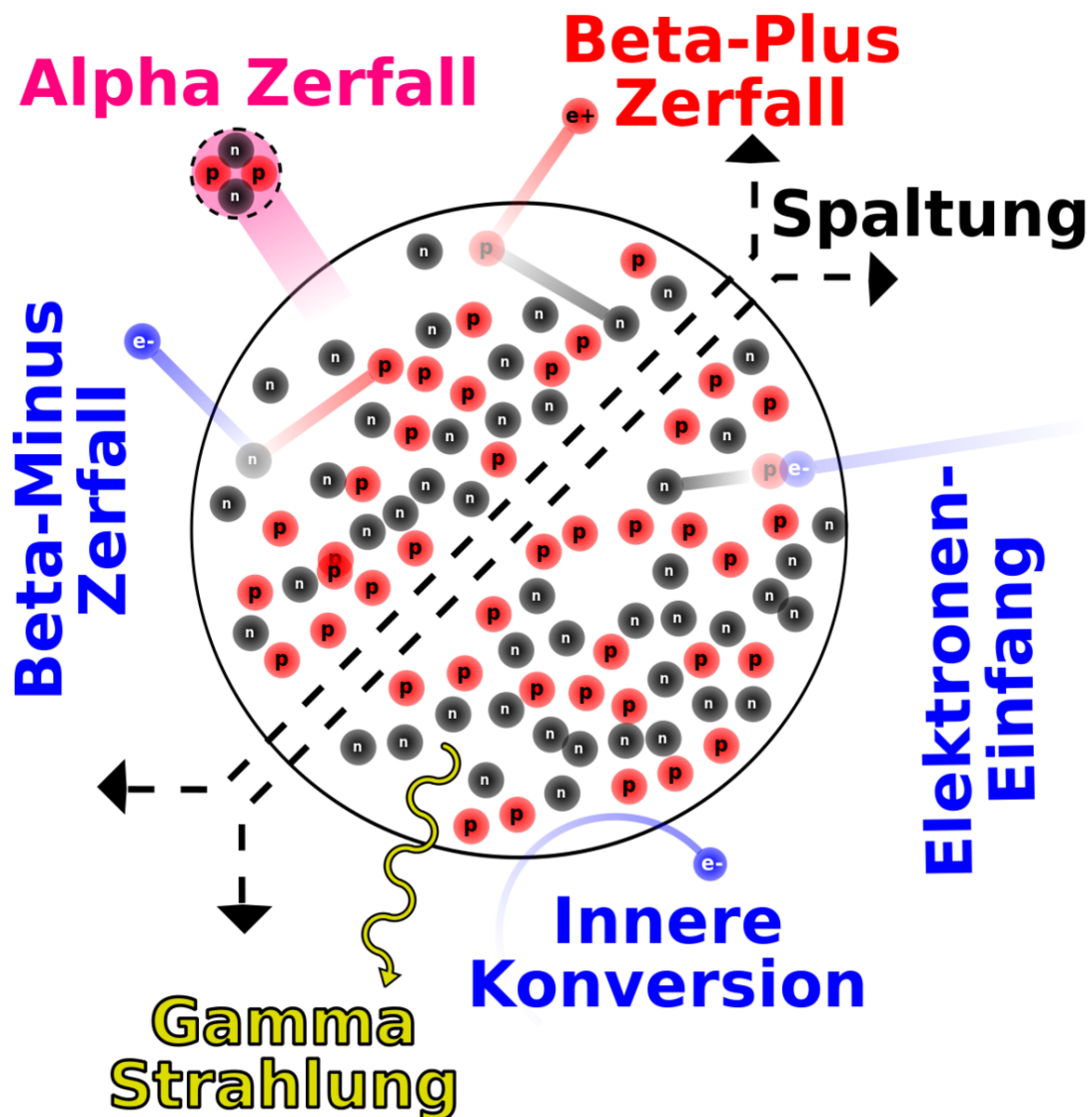
Abb. 3 Hypothetischer Kern, mit vielen Zerfallsmöglichkeiten
