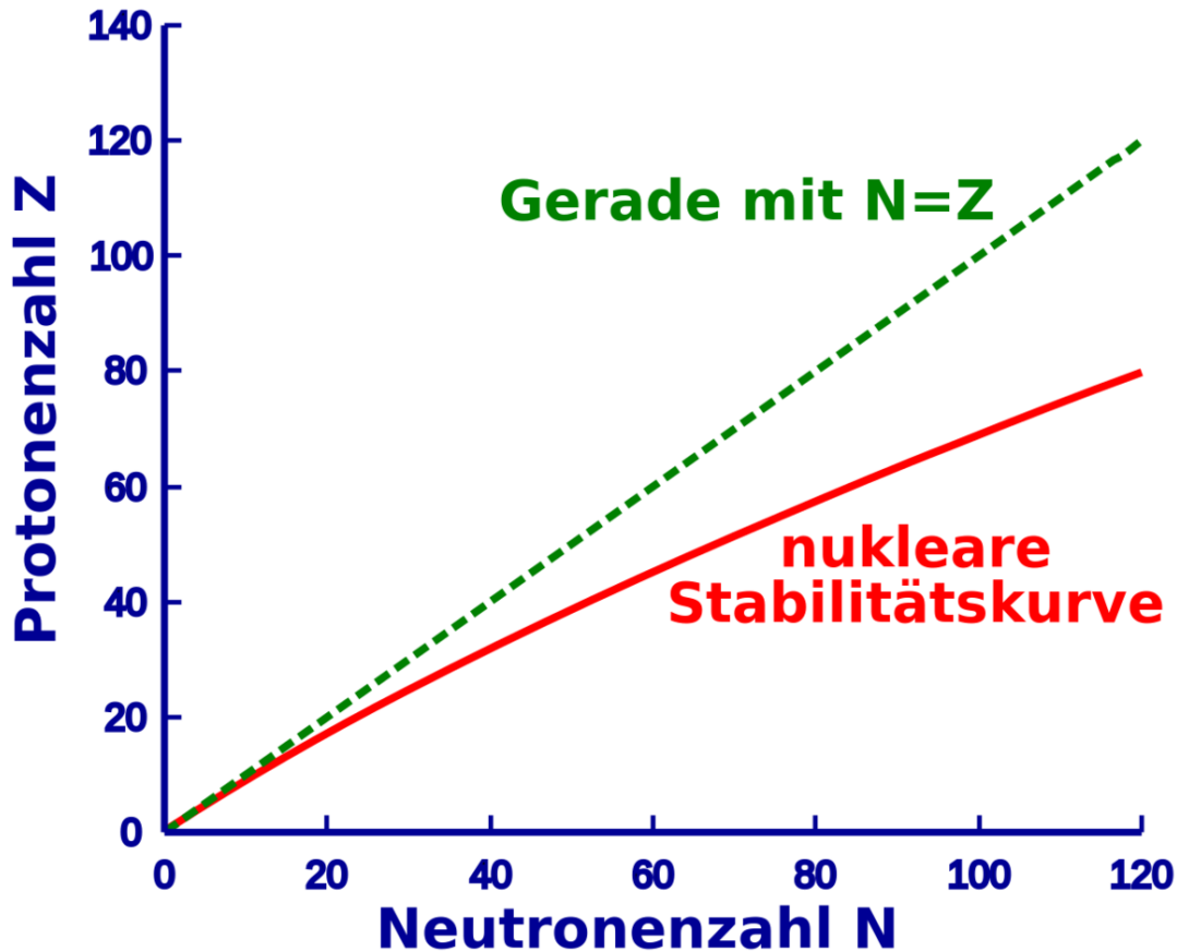
Abb. 2 Nukleare Stabilitätskurve
