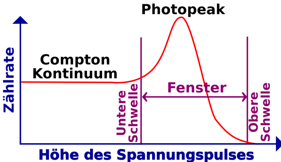
Abb. 49 Gammaspektrum mit eingezeichneten Diskriminatorschwellen
