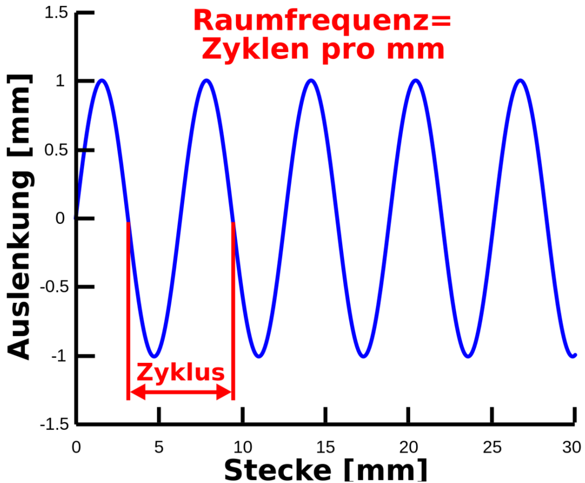
Abb. 132 räumlicher Verlauf einer Sinuswelle
