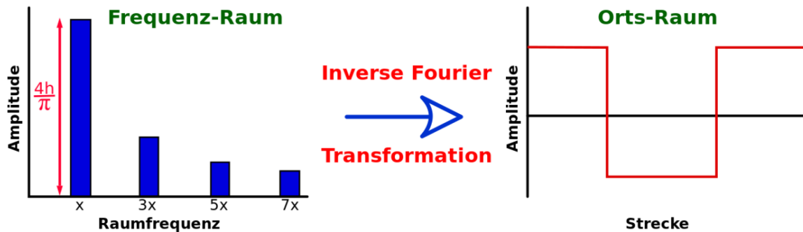
Abb. 147 Die inverse Fourier-Transformation kann verwendet werden um beliebige periodische Wellenformen beliebig genau anzunähern, wie hier am Beispiel der Rechteckfunktion gezeigt wird.
