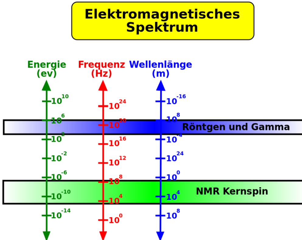
Abb. 4 Elektromagnetisches Spektrum
