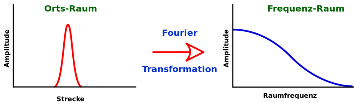
Abb. 149 Die Fourier Transformierte einer verbreiterten Delta Funktion.
