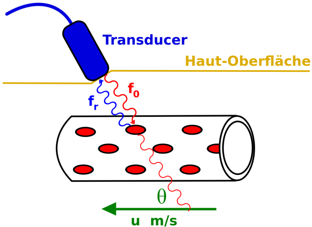
Abb. 175 Darstellung des Dopplereffekts
