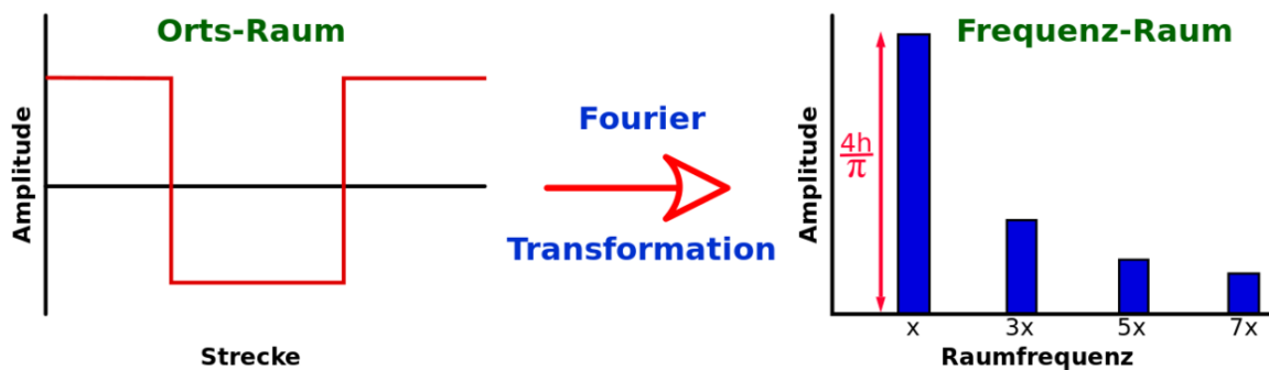
Abb. 146 Die Fourier-Transformation kann verwendet werden, um das Fourier-Spektrum jeder beliebigen Wellenform zu berechnen, wie hier am Beispiel der Rechteckfunktion gezeigt wird.
