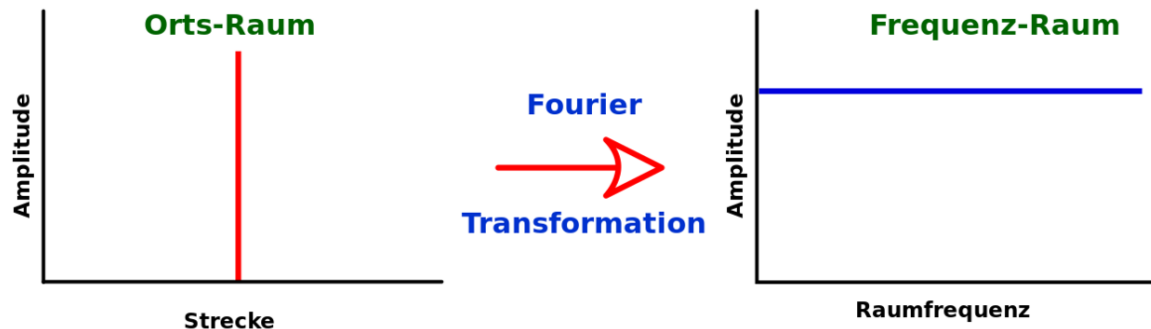
Abb. 148 Die Delta-Funktion (links) und ihre Fourier Transformierte (rechts)
