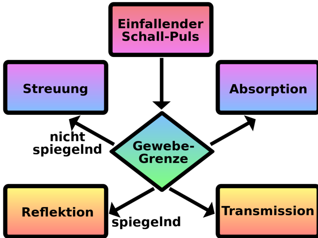
Abb. 161 Blockdiagramm einiger Wechselwirkungen akustischer Wellen mit einer Grenzfläche zweier Gewebe
