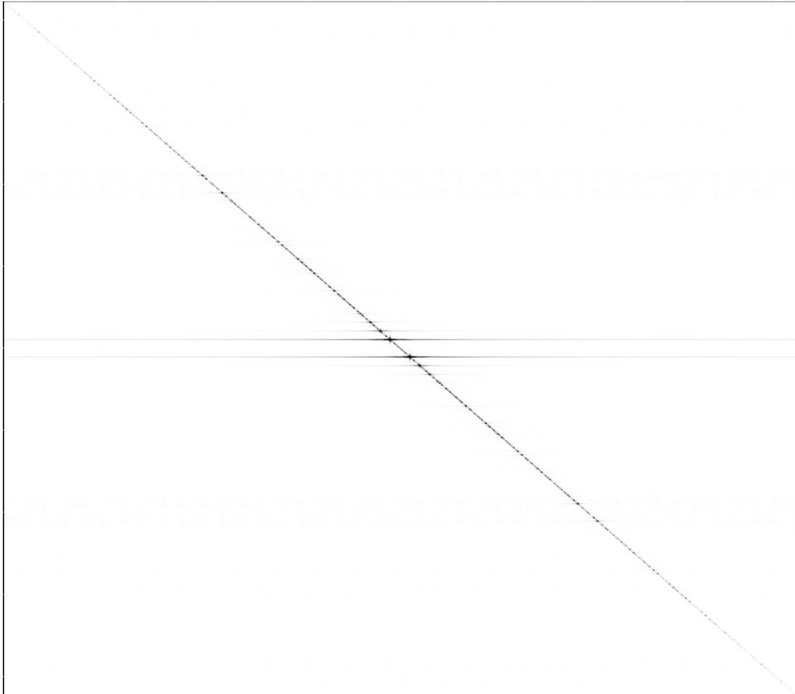
Abb. 128 (d) die 2 dimensionale Fouriertransformation von (a)
