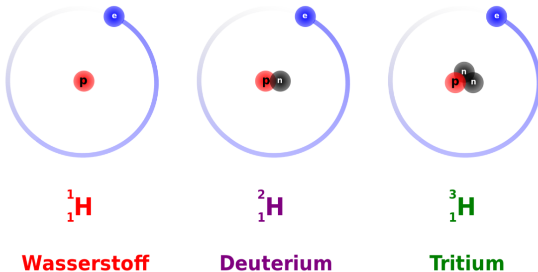
Abb. 1 Schematische Darstellung der Atome: Wasserstoff, Deuterium, Tritium
