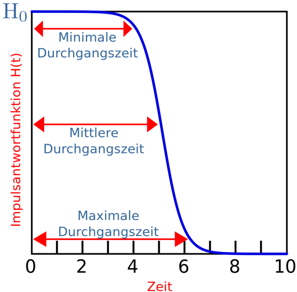
Abb. 157 Allgemeine Form der Impulsantwortfunktion die sich bei einer Entfaltungsrenographie ergibt
