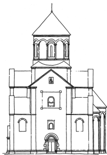
Свято-Пантелеймонівська церква. Західний фасад. Реконструкція І. Могитича.
