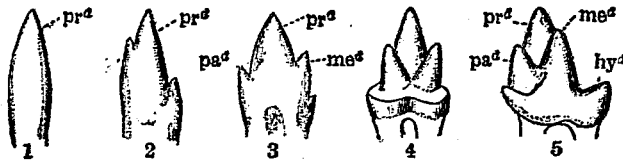
第二十二圖 原始哺乳類之齒之進化
