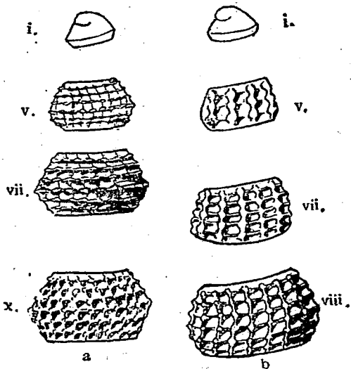
第九圖 兩種 Procerithium 之 homœomorphy
