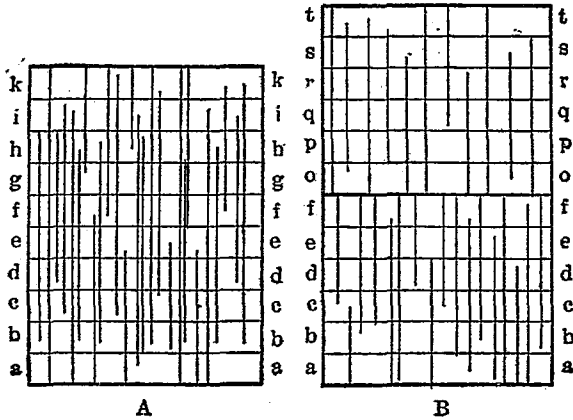
第十一圖 地質時代之間隙 (據 Marr)
