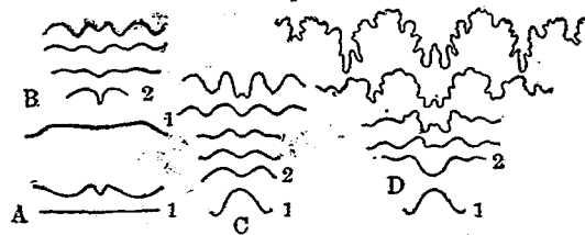
第十圖 菊石類縫合線之發達
