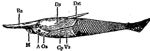
第二十圖 Pteraspis 之復舊圖 (據 Abel)
