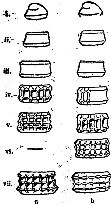
第八圖 英國侏羅紀之 Procerithium 之螺層發達之比較 a 為 P. ogerieni b 為 P. numismale (據 Mc Donald 與 Trueman)
