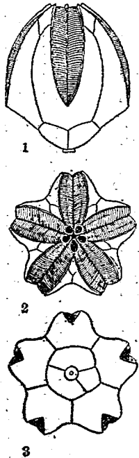
第十六圖 Pentamerites （海蕾類之例） 1 由橫視； 2 由上視； 3 由下視。
