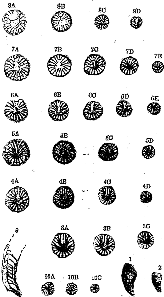
第七圖 Zaphrentis delanoyei 之進化 (二倍半)
