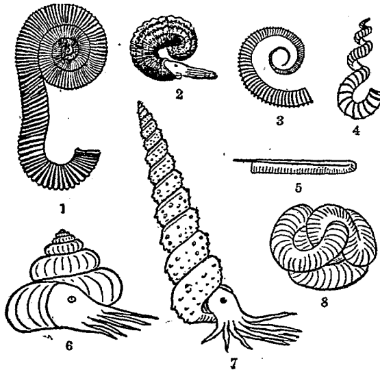
第十四圖 種種菊石類之形狀
