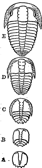
第六圖 Suo hirsuta 之發達
