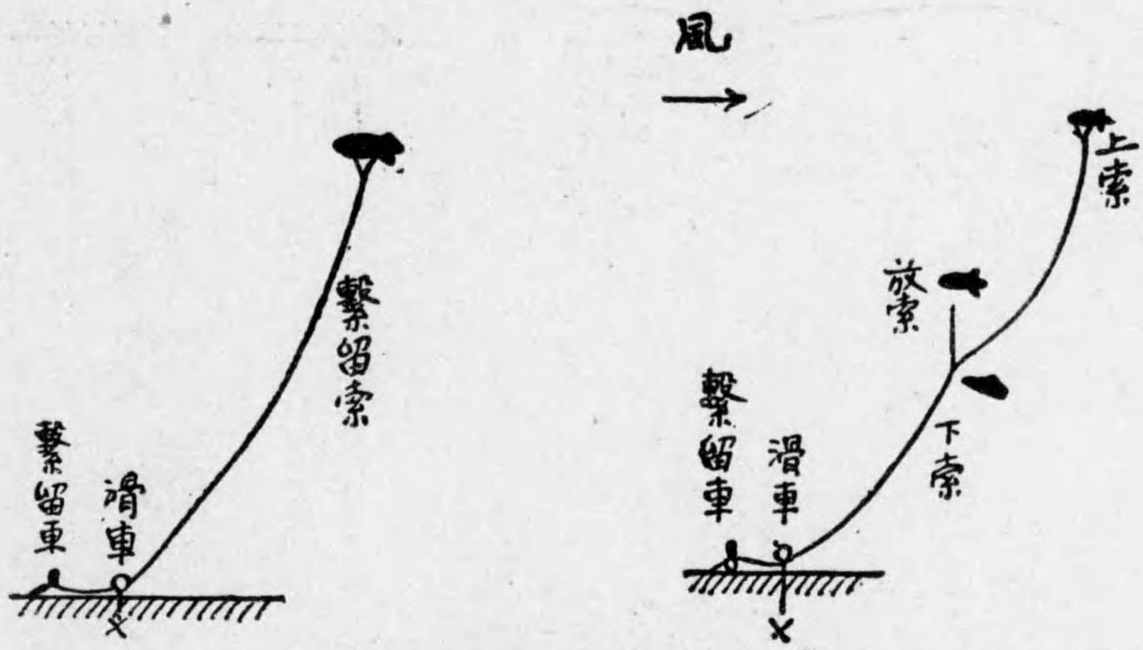
ルターメ千四とだ式(複式) 球氣式(單式)は左、球氣式(複式)は右 き大てしと球氣空防 でのる來出がとこるげ揚く高も (る來出がとこす果を 目役な
