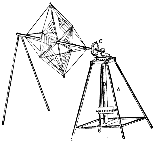
車 風 小
