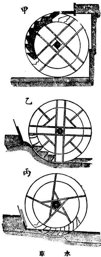
車水 (甲)上射水車 (乙)中射水車 (丙)下射水車
