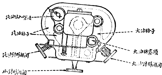
氣化器
