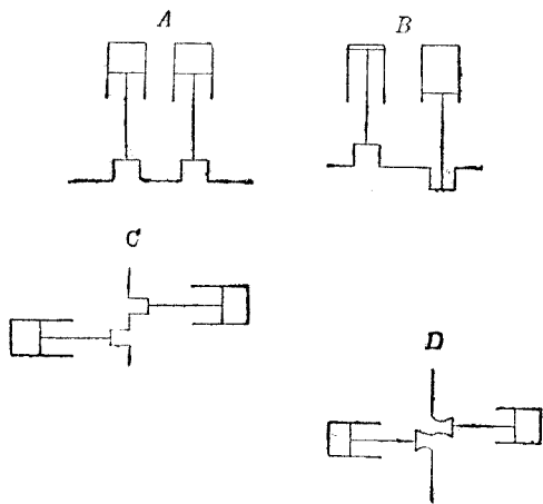
第五十四圖
