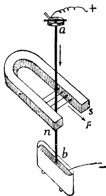
圖九十六第
