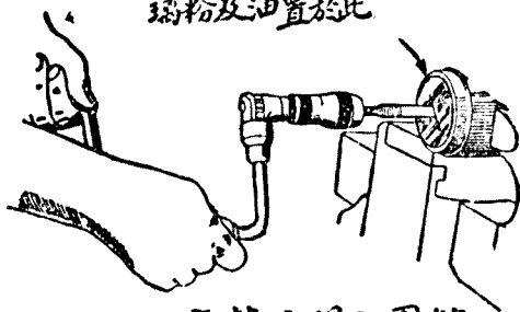
解圖之活門整磨
