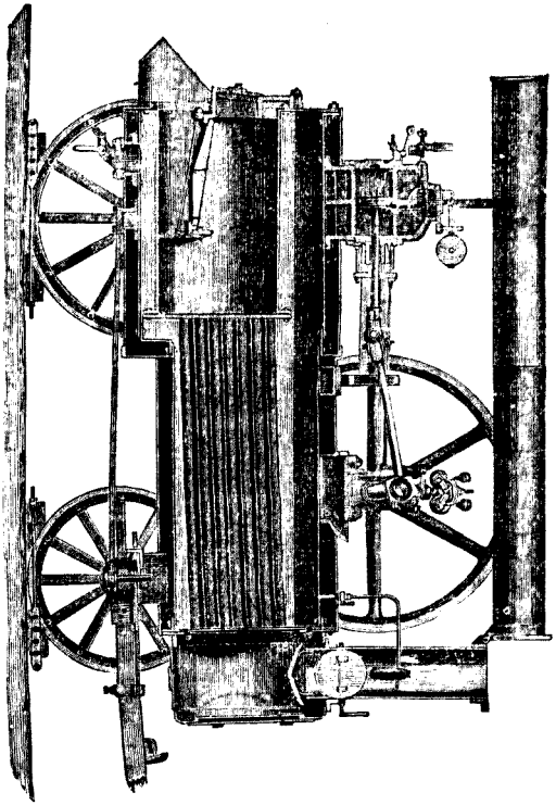
蒸汽助引機
