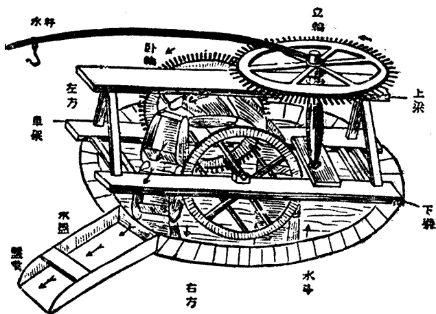
水車全部
