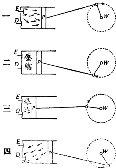
圖一十五第
