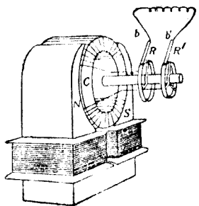
圖十七第
