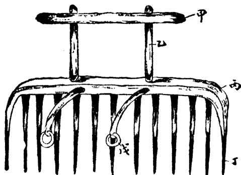
耙 字 而
