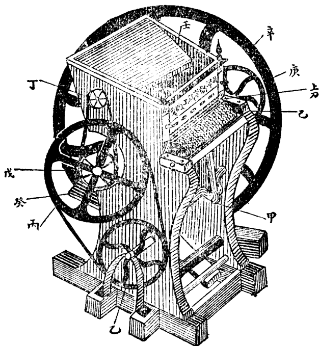
機 棉 軋 軸 鞞
