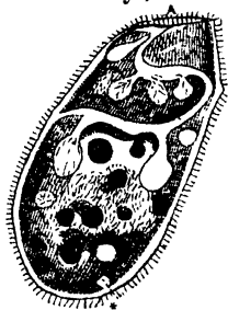
Fig. 171.— Leucophrys patula .
