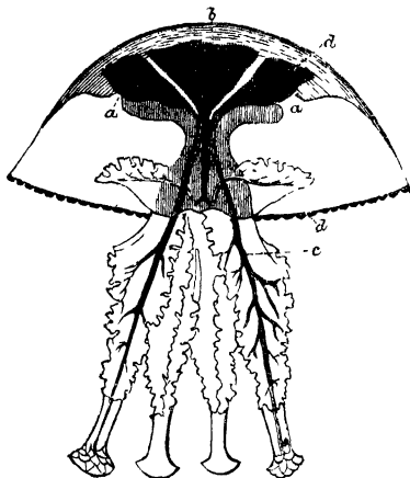
Fig. 173.— Rhizostoma Cuvieri .
