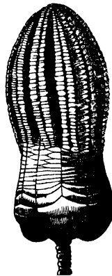
Fig. 73.— Encrinurus moniliformis .
