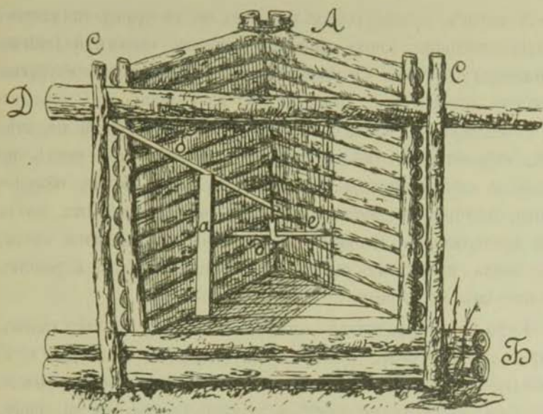
Фиг. 6. Кулема.
