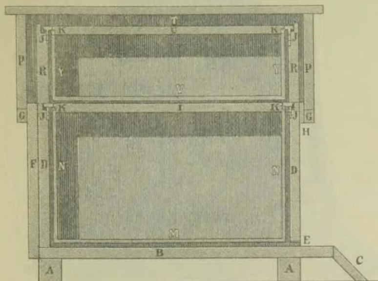
Фиг. 1. Улей Лангстратъ-Дадана въ вертикальномъ разрѣзѣ.
