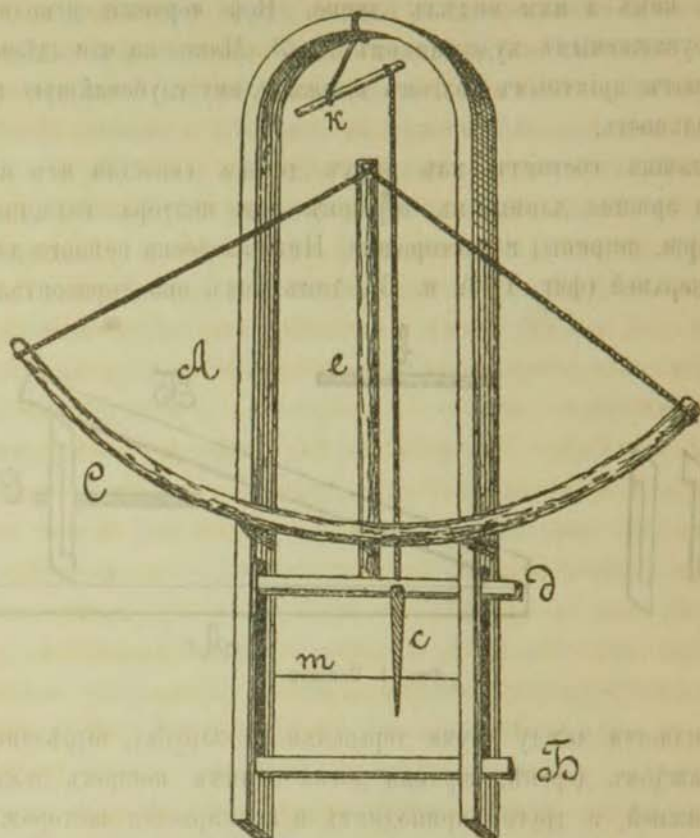
Фиг. 2. Черкань.
