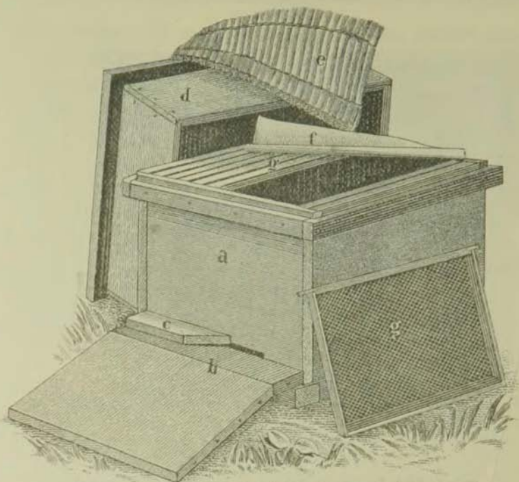
Фиг. 2. Улей Лангстротъ-Дадана, открытый.
