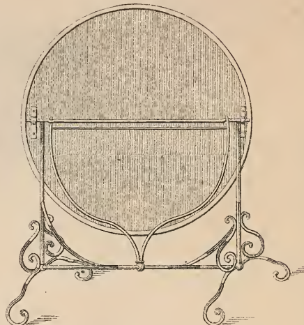
N°5 fixe, ronde
