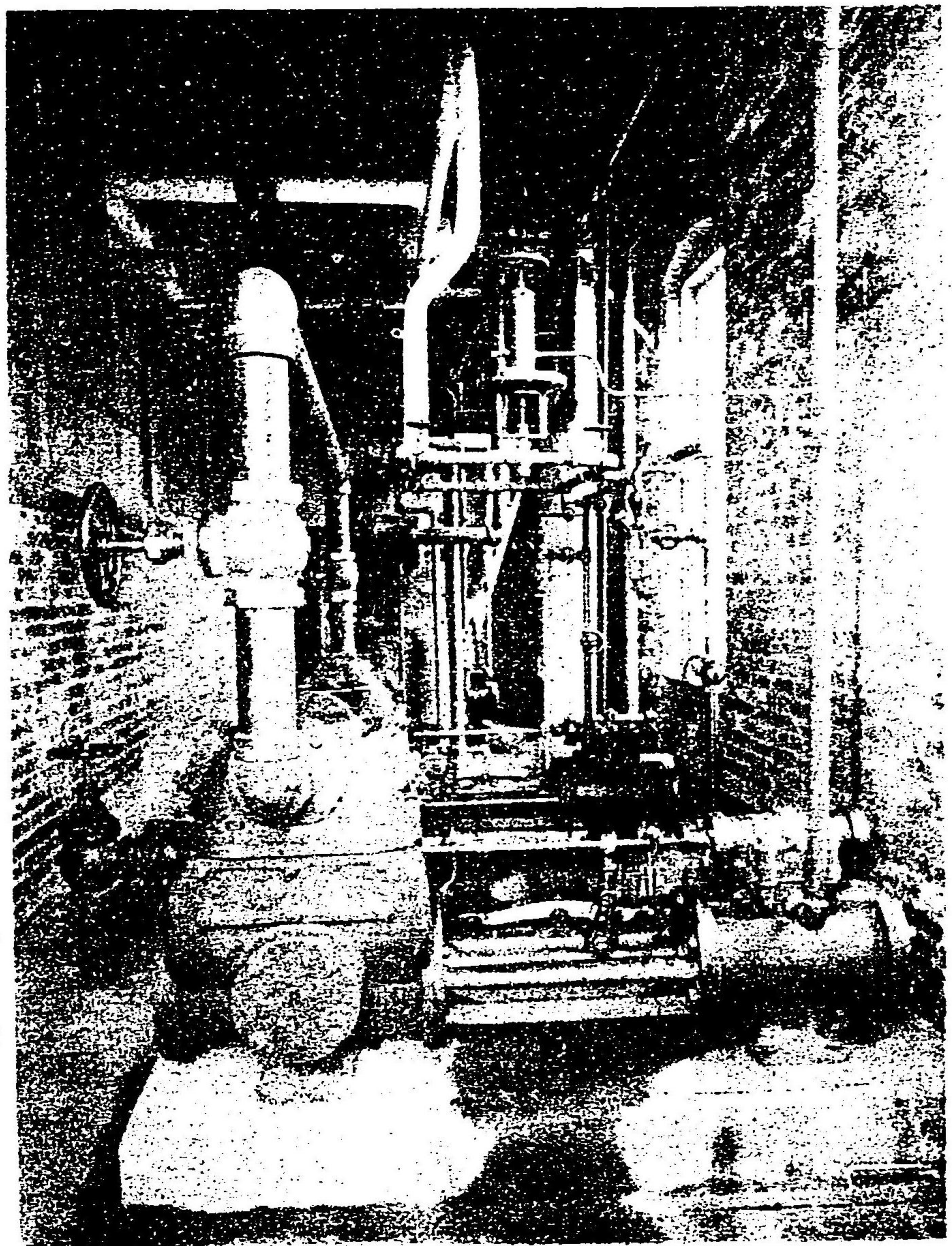
ウエブスター式低壓蒸氣暖房裝置
