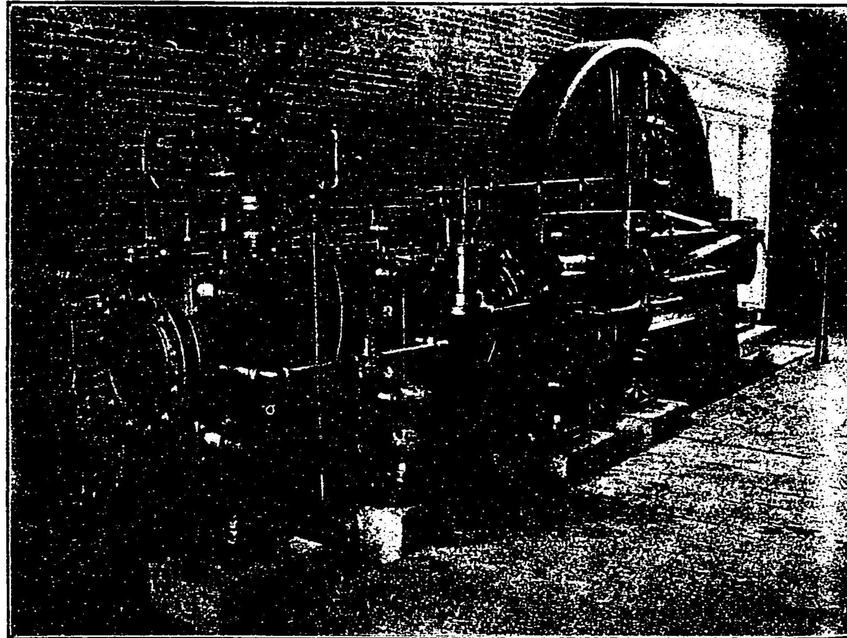
(一其) 壹百貳拾馬力蒸汽機關 (中島三工所製)
