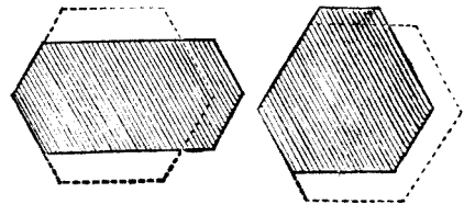
第四十三圖 面角之安定
