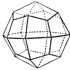
五第十四圖 偏斜方三八面體
