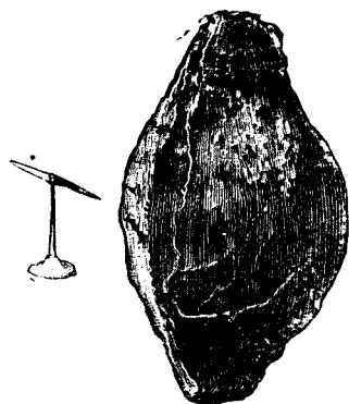
火山彈
