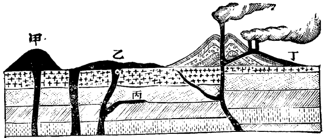
第 九 十 六 圖 火 山
