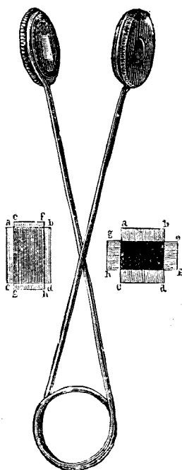
第八十一圖 電氣石鏡
