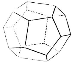
第五十七圖 五角十二面體
