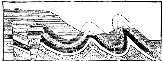
斷 層 向 斜 背 斜
