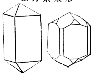
正方系聚形
