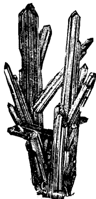
輝銻礦
