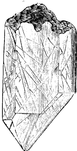
第二十二圖 草入水晶
