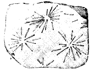
第三十七圖 電氣石
