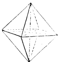
第一正方錐
