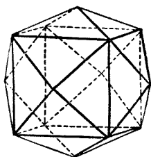
五第十二圖 四六面體
