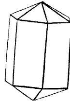
第六十四圖 六方系聚形
