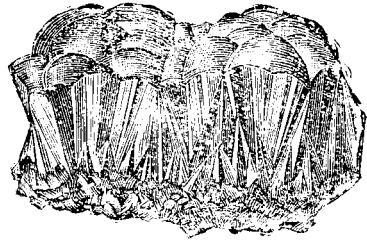
赤鐵礦
