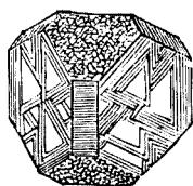
第十六圖 閃鋅礦
