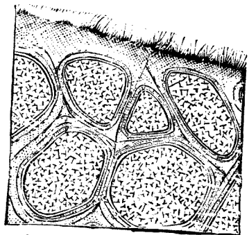
花崗巖之風化
