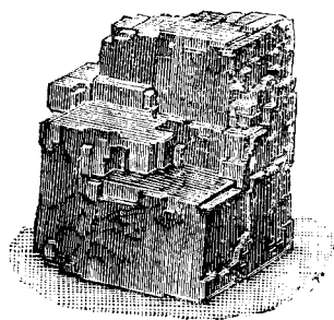
方鉛礦
