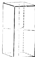
第一正方柱
