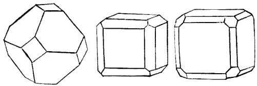
第五十八圖 等軸系聚形
