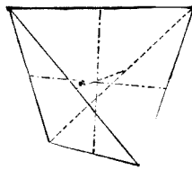
第五十六圖 四面體
