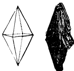
第四十二圖 硫黃結晶
