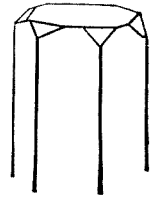
第六十四圖 六方系聚形
