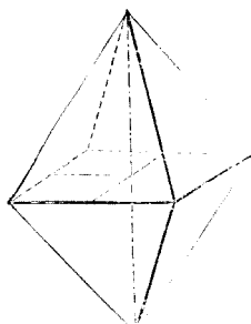
第二正方錐
