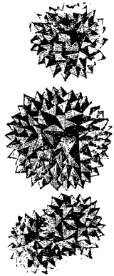
第二十圖 自然砒
