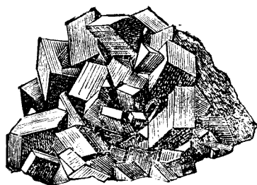
菱鐵礦
