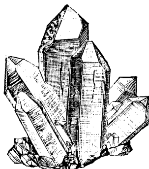
第二十一圖 水晶之晶羣
