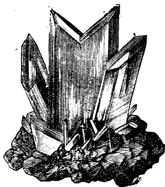
第三十二圖 石膏
