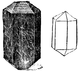
第三十六圖 磷灰石
