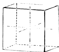
六面體
