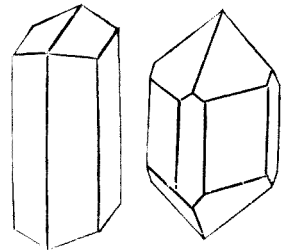
單斜系聚形
