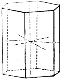
第六十三圖 第二六方柱
