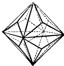
五第十三圖 三角三八面體
