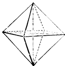
八面體
