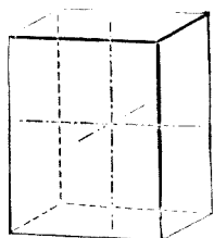
第二正方柱
