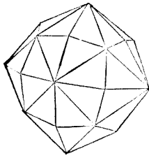
第五十五圖 六八面體
