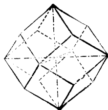
斜方十二面體
