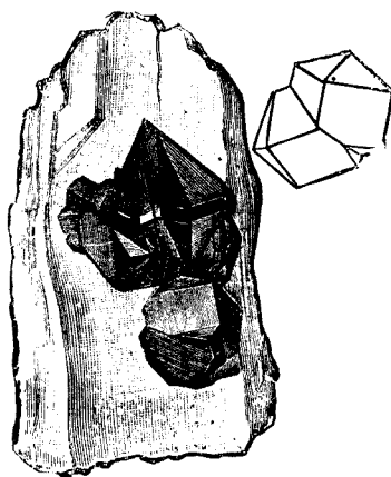
第十七圖 錫石
