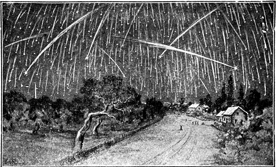
一八三三年十一月十三日美國各地衆星下壓之情形
