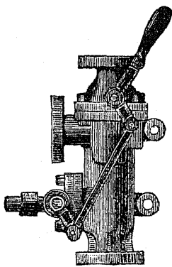
Универс. Инжекторъ.
