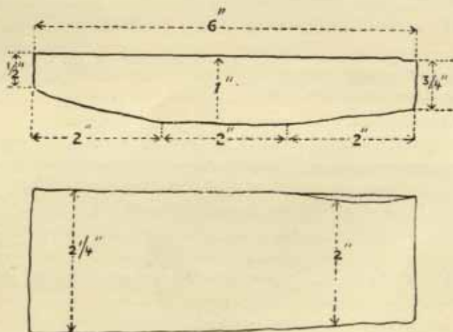
Fig. 2 Blooms in Konarak Iron.
