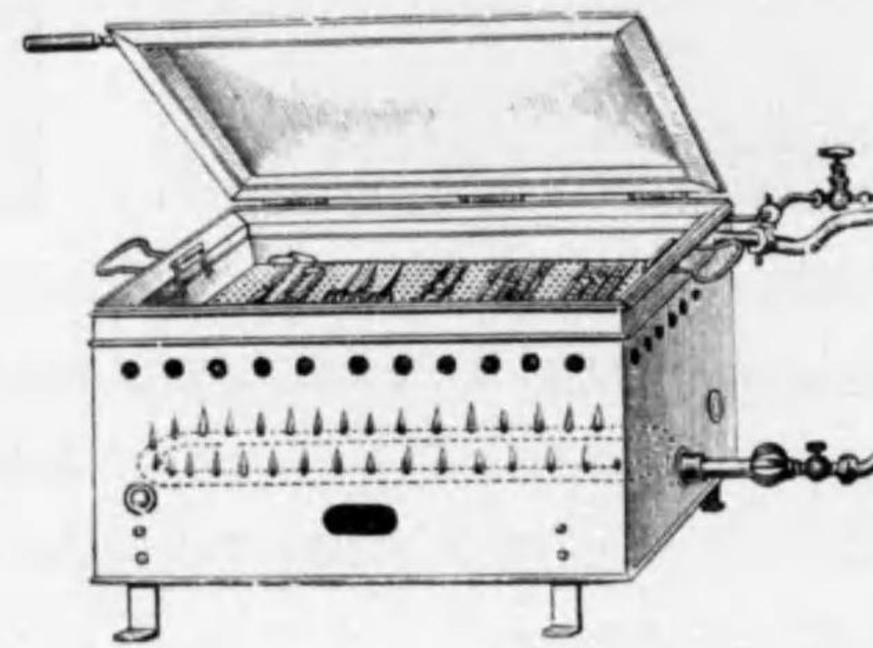
シムメルブッシュ氏器械消毒器
