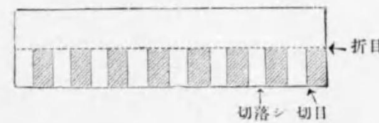
第四百三十五圖 有窓義布斯繃帶用厚紙(甲)
