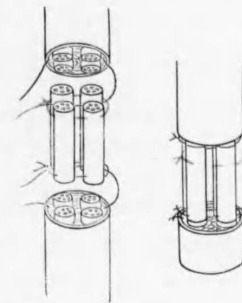
神經挿入移植法 (n. Lehmann)
