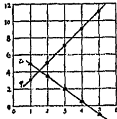
圖 6-1. 完全相關.
