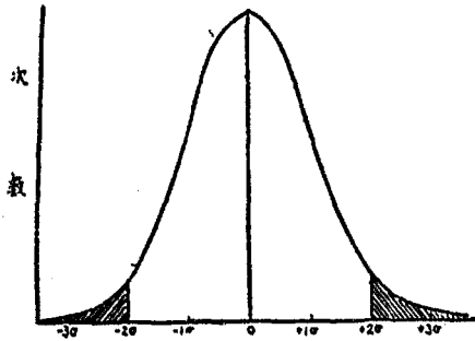
圖 7-4. 常態曲線圖
