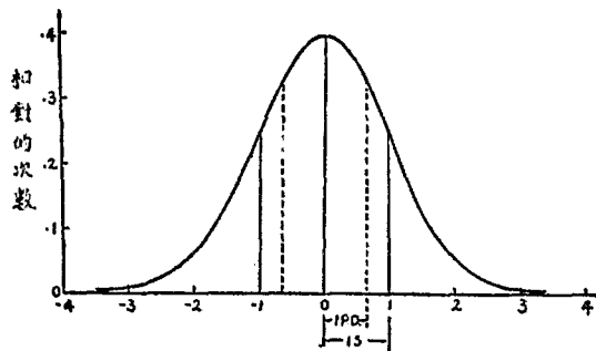
圖 4-4. 常態曲線圖。
