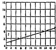
圖 6-2. r=0.91 .
