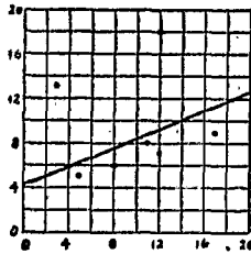
圖 6-3. r=0.40 .
