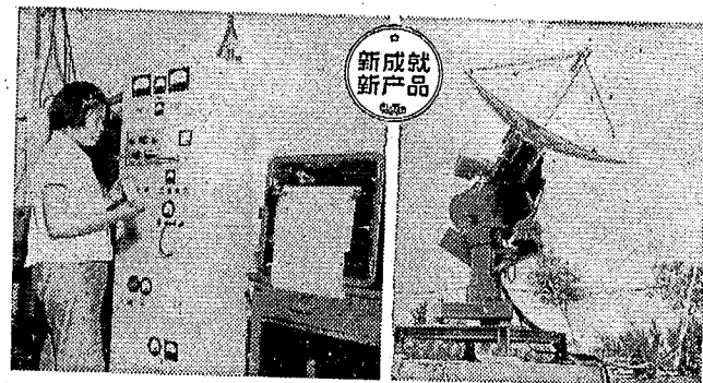
左图是太阳射电望远镜接收机正在把从太阳上发出的微波放大并自动记录下来。右图是太阳射电望远镜的天线微波自动跟踪系统。（新华社记者姚文摄）
