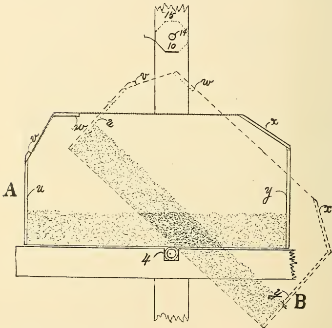
FIG. 73. USING THE TILT BOX.
