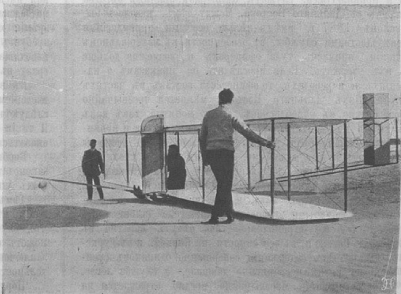
Бипланъ Райта безъ двигателя.
