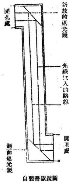
自製潛望鏡圖
