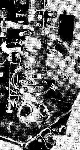
我国第一台一级大型电子显微镜在上海试制成功。这台显微镜的放大倍数最大为二十万倍，分辨本领达到七埃。它是由我国科学技术人员和工人自行设计、自行制造、全部采用国产原材料制成的。
