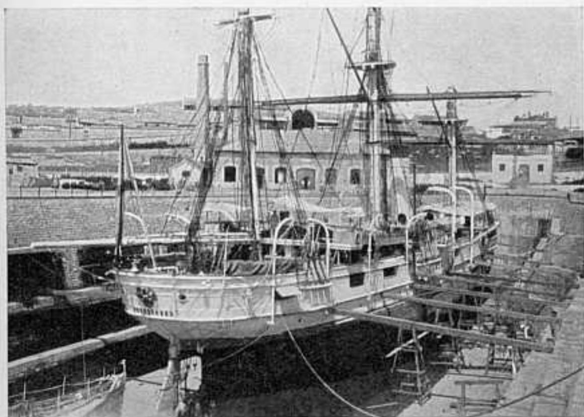
ВНУТРЕННИЙ СУХОЙ ДОКЪ ВЪ ПОРТЪ-АРТУРЪ.
