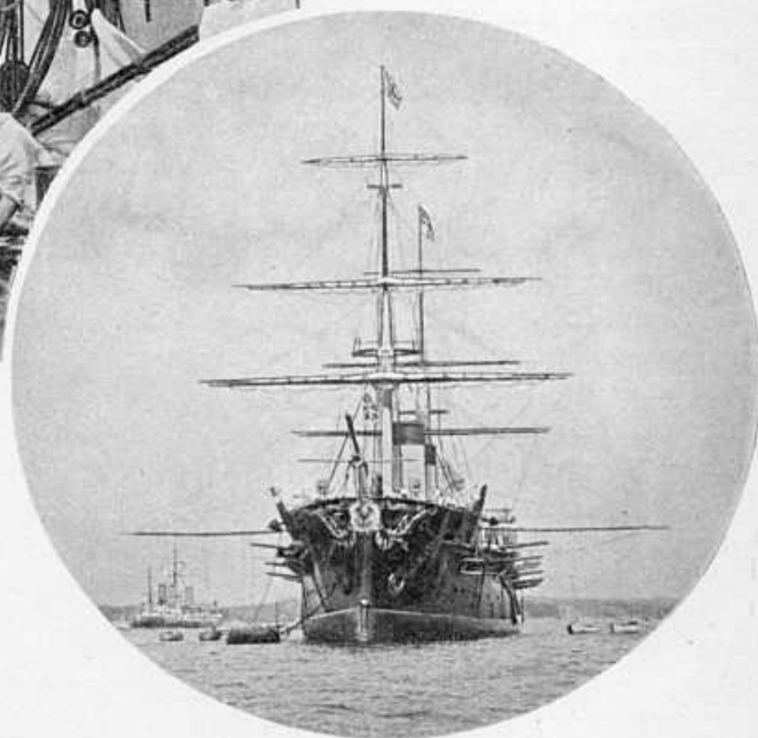
БРОНЕНОСНЫЙ КРЕЙСЕРЪ 1-ГО РАНГА «РЮРИКЪ».
