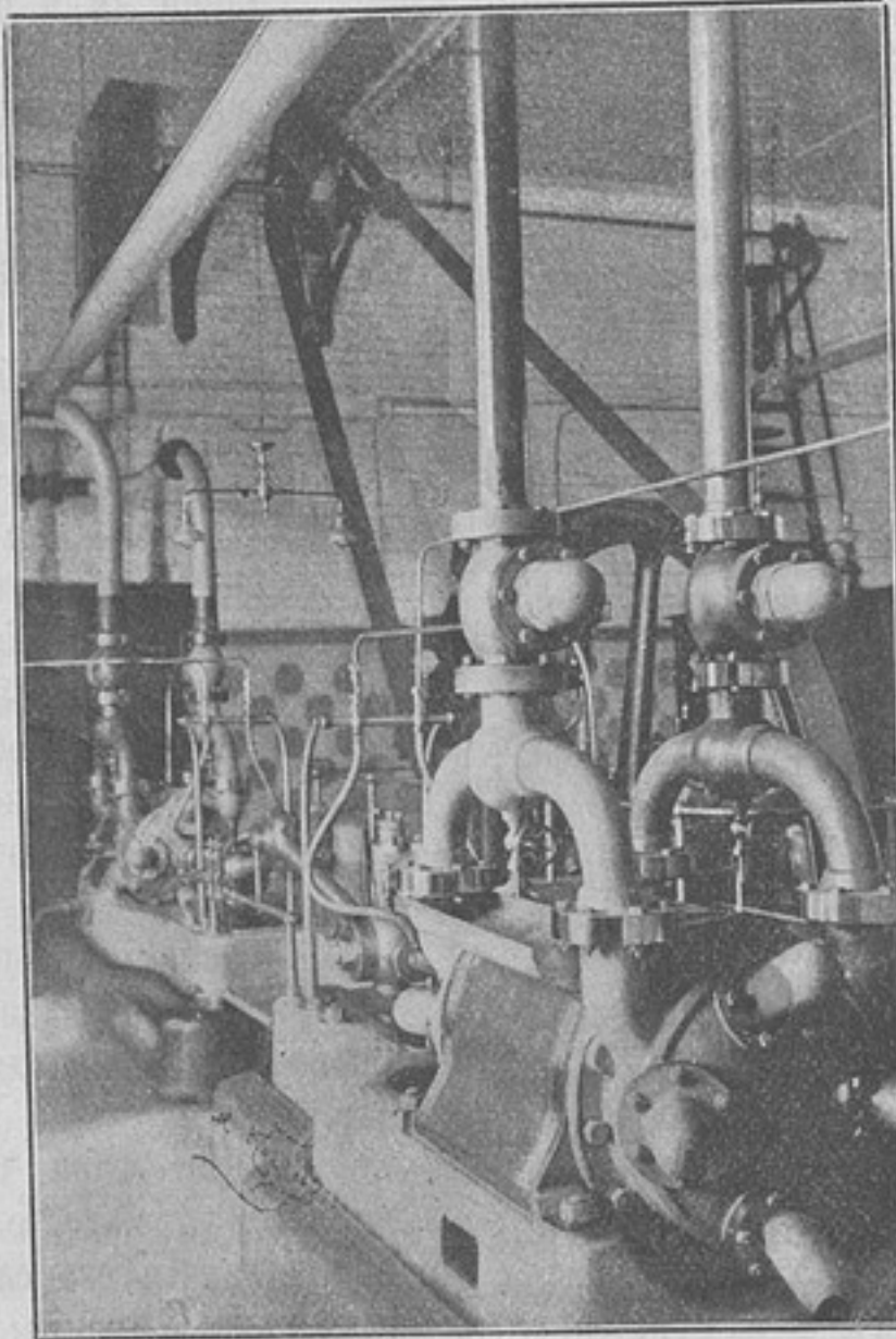
Машина (Frigorifer) системы «Рауля Пиктета» для полученія искусственнаго холода (къ статьѣ «Соображенія объ употребленіи искусственно-замороженной рыбы, для временнаго продовольствія войскъ въ крѣпостяхъ»).
