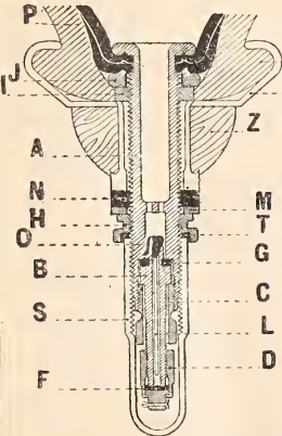
COUPE DE LA VALVE VOITURE Modèle 1903.
