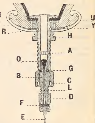
COUPE DE LA VALVE "TERMINUS" Modèle 1898.
