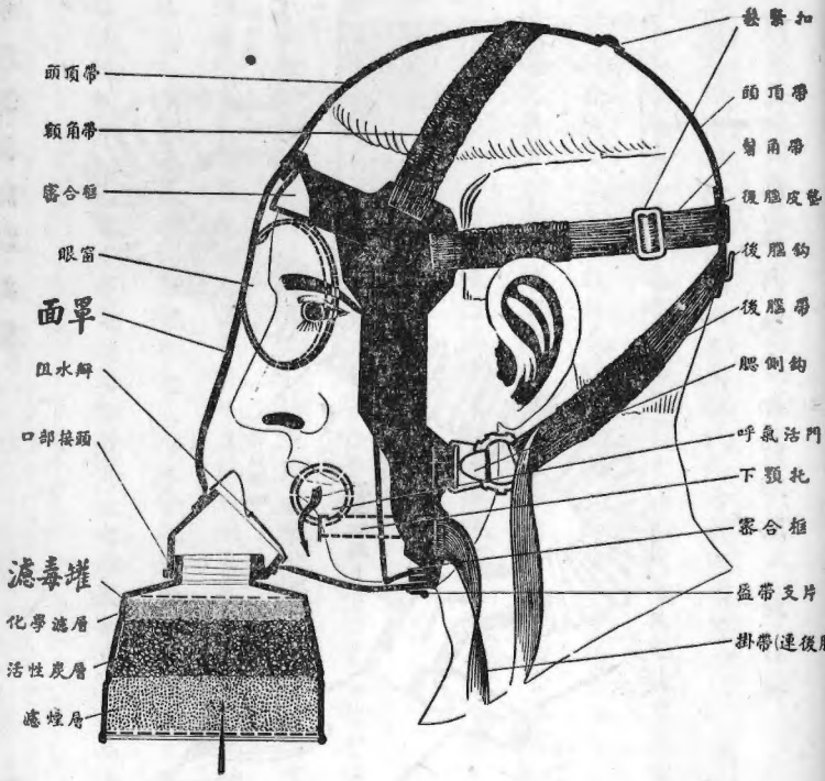
稱名之部各具面毒防 圖一第
