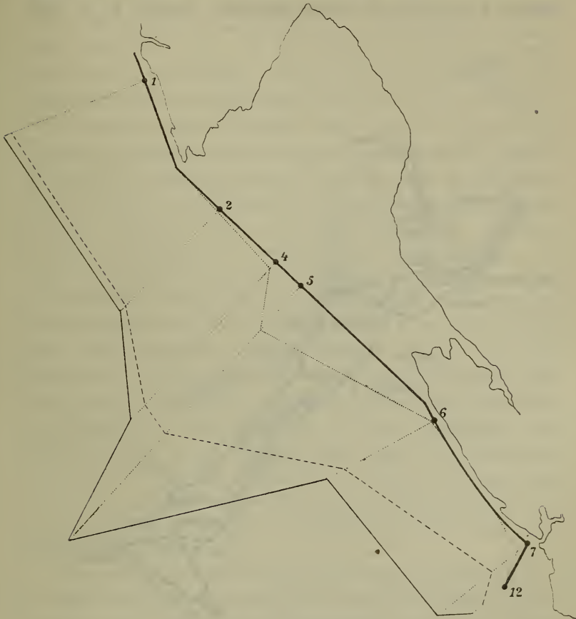
Fig. 2. Planktonkurve.
