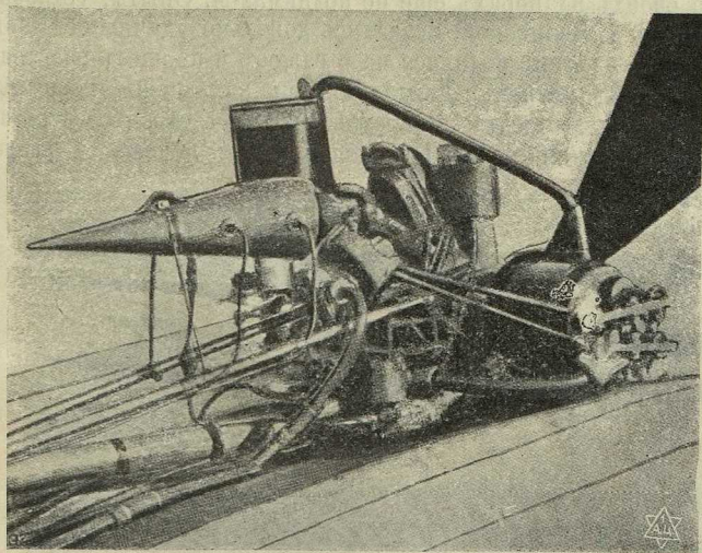
Моторъ аэроплана „Demoiselle“ (видъ сзади).
