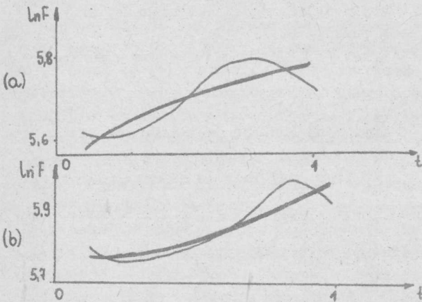
Rys. 2. Aproxymacja przebiegów częstotliwości podstawowej
