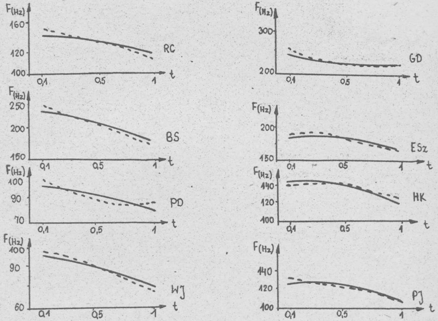
Ryc. 5. Przebiegi częstotliwości podstawowej i ich aproksymacje w zdaniu "lech nie wytrzepał" b/ sylaba "trze".
