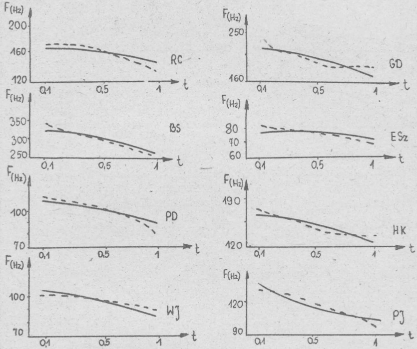
Ryc. 6. Przebiegi częstotliwości podstawowej i ich aproksymacje w zdaniu "lech nie wytrząpał go dziś" b/ sylaba "trze".
