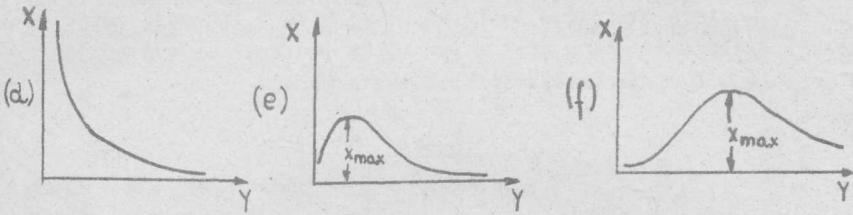
Rys. 1. Wykresy funkcji x = ay^b e^{cy} .
