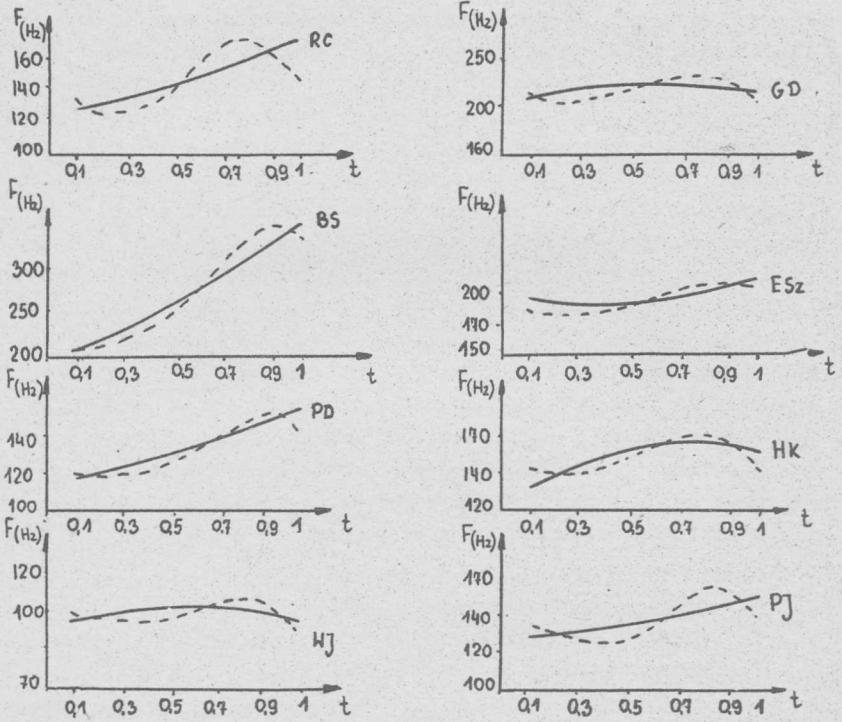
Ryc. 3. Przebiegi częstotliwości podstawowej i ich aproksymacje w zdaniu "lech trze". Funkcję aproksymującą zaznaczono linią ciągłą a/ sylaba "lech".
