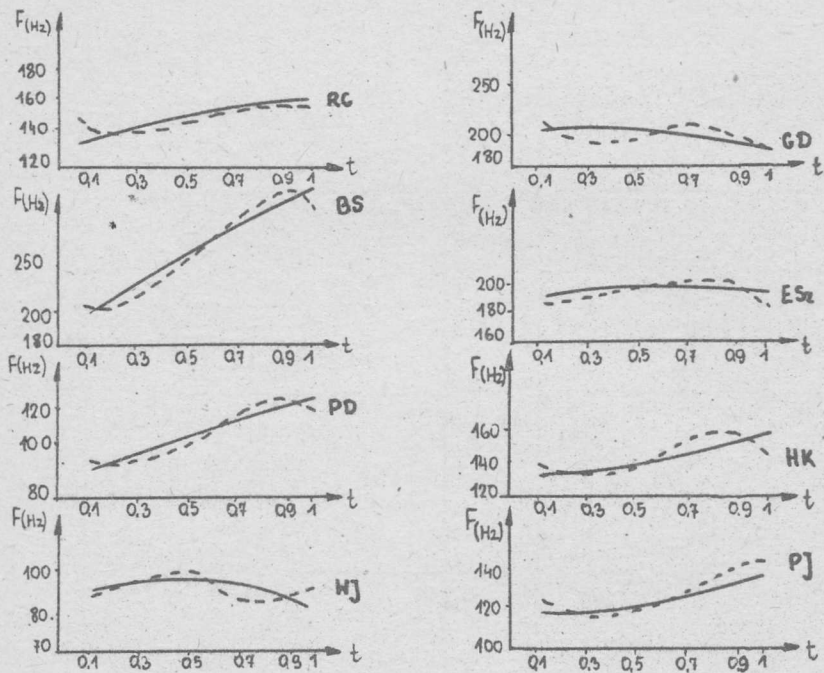
Ryc. 4. Przebiegi częstotliwości podstawowej i ich aproksymacje w zdaniu "lech wytrze" a/ sylaba "lech".
