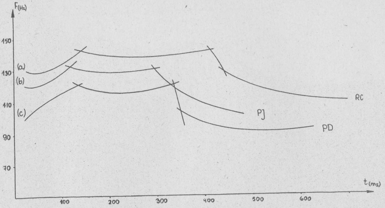
Ryc. 8. Aproksymacje przebiegów częstotliwości podstawowej w zdaniu "lech wytrzepał go" a/ głos PD b/ głos PJ c/ głos RC Aproksymacji dokonano na sylabach akcentowanych, między nimi oraz na sylabach końcowych.
