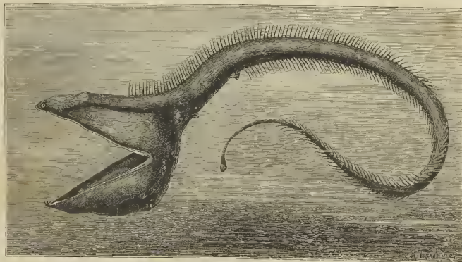
EL EURIPHARINX PELECANOIDES, nuevo pez de las profundidades del Atlantico.
