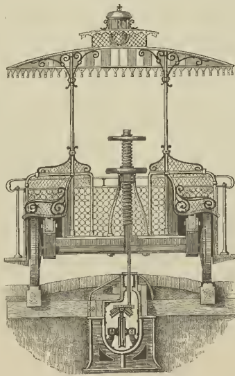
VISTA DE FRENTE DEL COCHE-GUIA Y SECCION TRASVERSAL DEL TUBO POR DONDE CORRE EL CABLE METÁLICO
