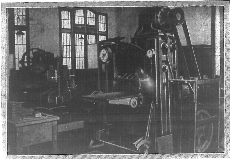
電 鍍 銅 版 部 壓 版 機
