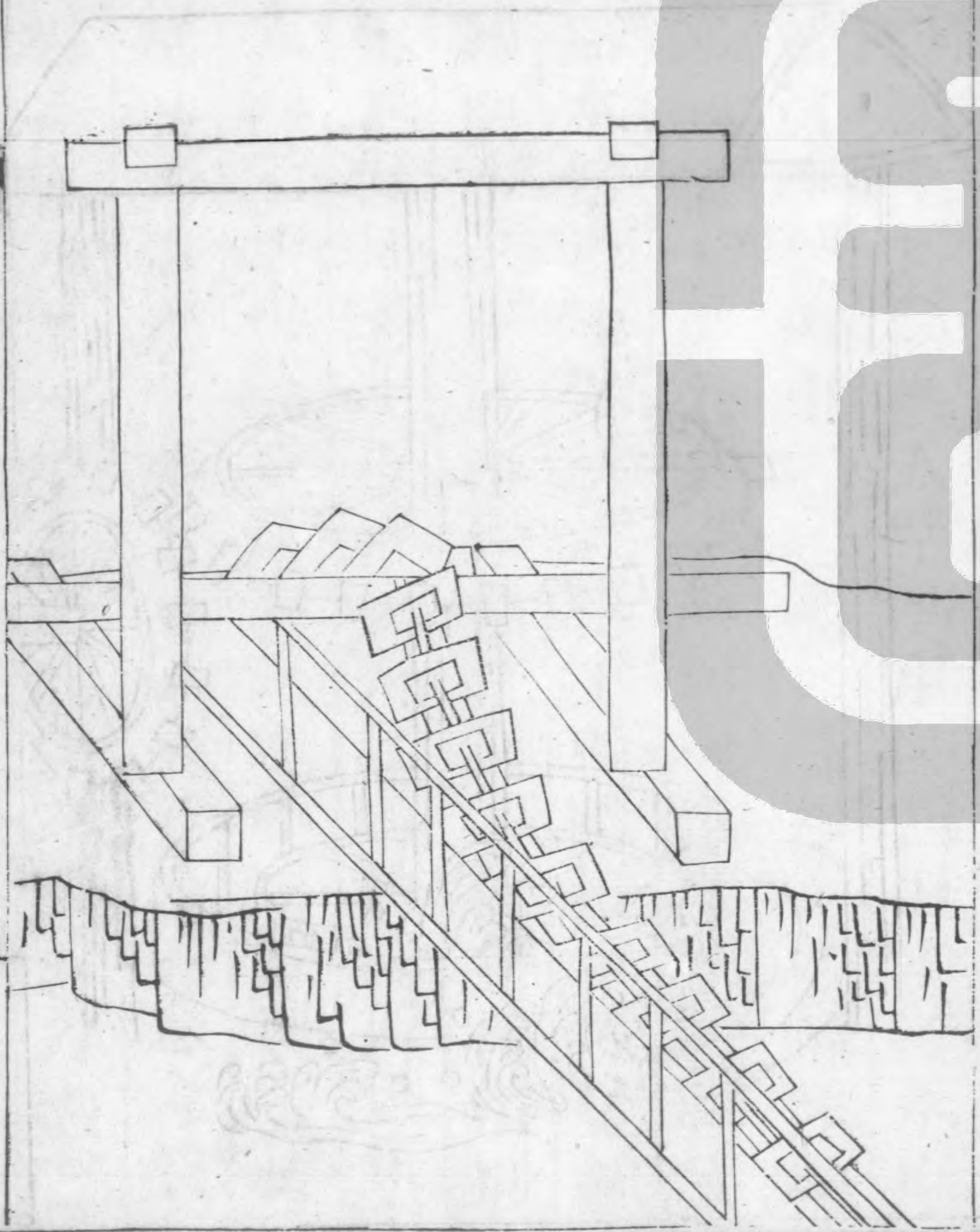
水轉翻車
