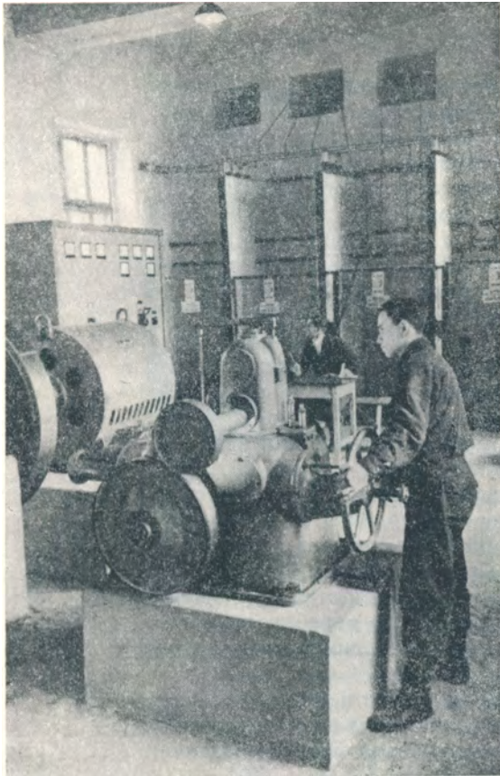
Машинний зал Міліївської електростанції. 1952 р.
