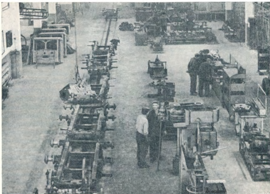
У ремонтній майстерні райоб'єднання «Сільгосптехніка», с. Веренчанка, 1968 р.
