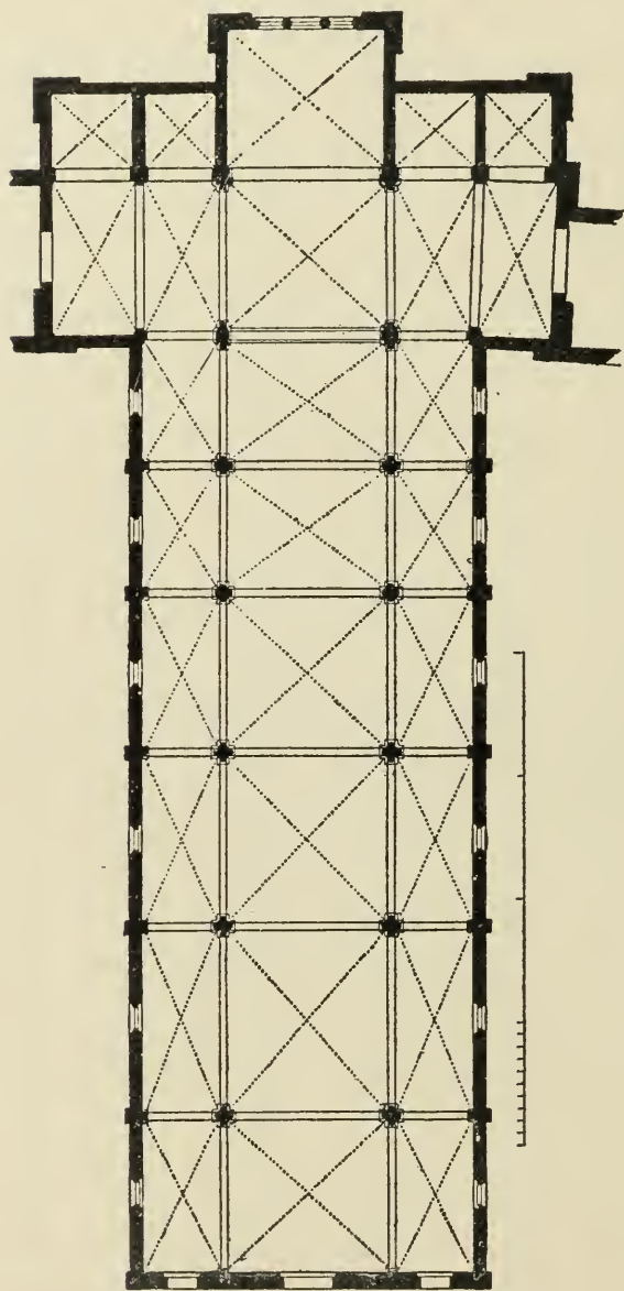
Fig. 348. Florence. S. M. Novella.
