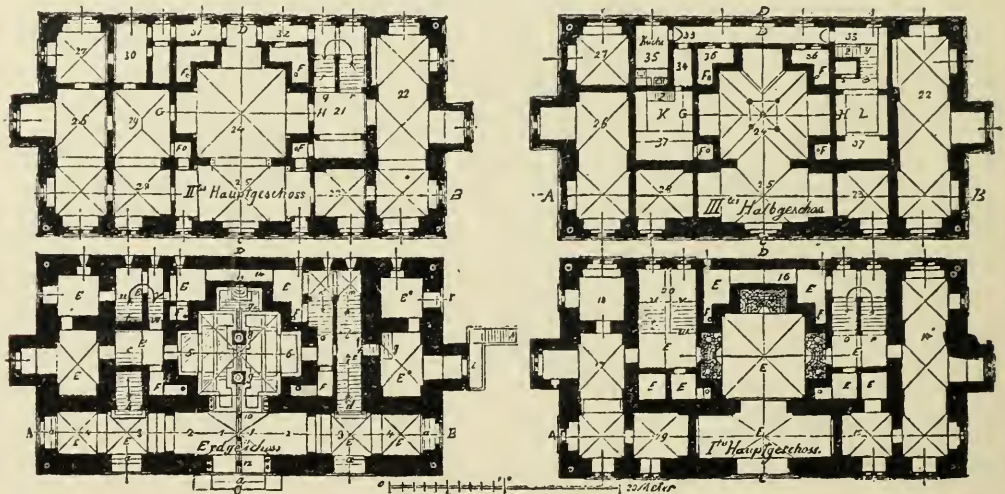
Fig. 319. Palermo. Story Plans of La Zisa.
