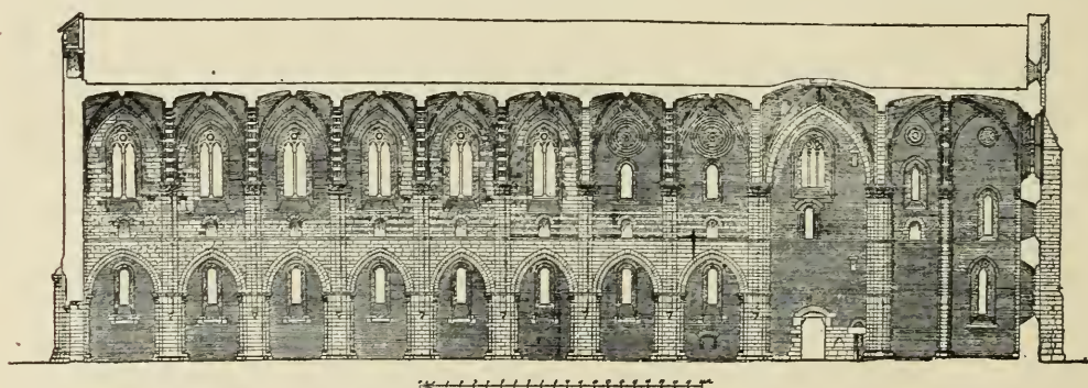
Fig. 336. S. Galgano. Section.
