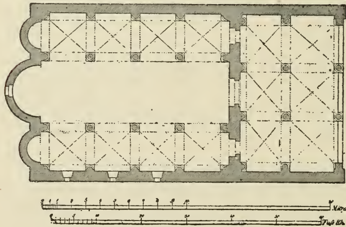
Fig. 270. Trani. Ognissanti.
