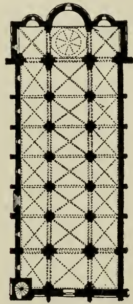
Fig. 340. Barletta. S. Sepolcro.
