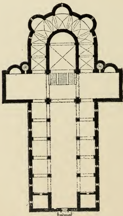
Fig. 262. Acerenza Cathedral.
