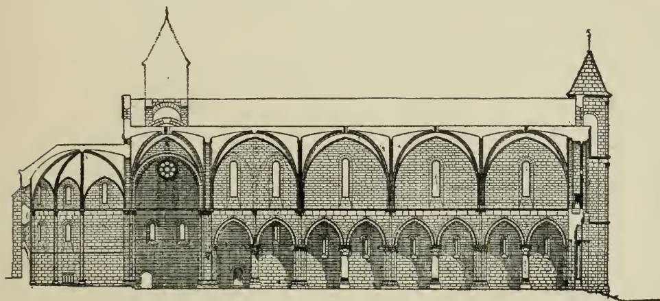
Fig. 339. S. Martino. Longitudinal Section.
