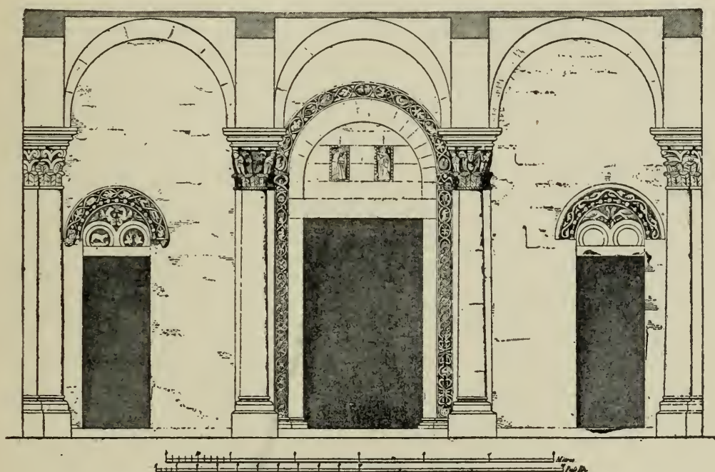
Fig. 271. Ognissanti. Section of Porch.
