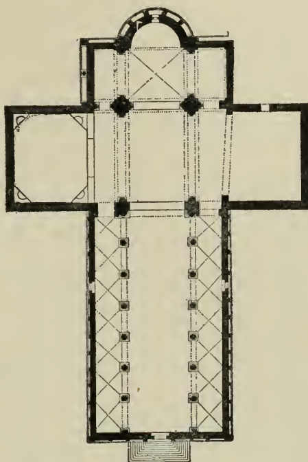
Fig. 254. Troja. Cathedral.
