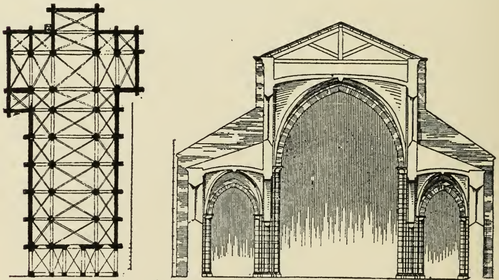
Fig. 327. Chiaravalle di Castagnola. Plan and Section.
