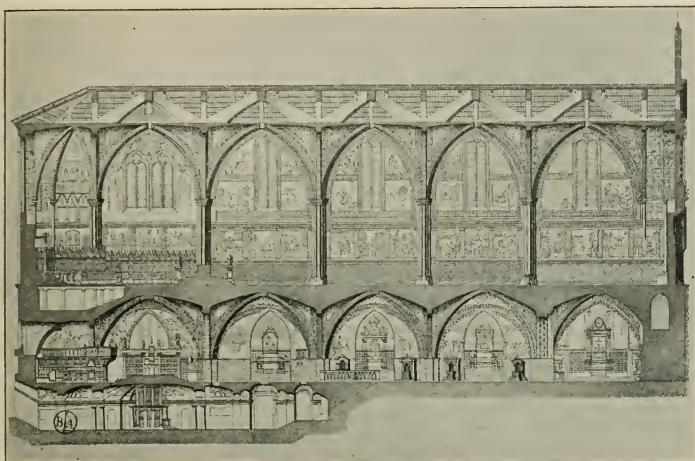
Fig. 343. Assisi. Longitudinal Section of S. Francesco.
