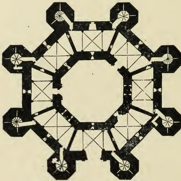
Fig. 404. Plan of Castel del Monte.
