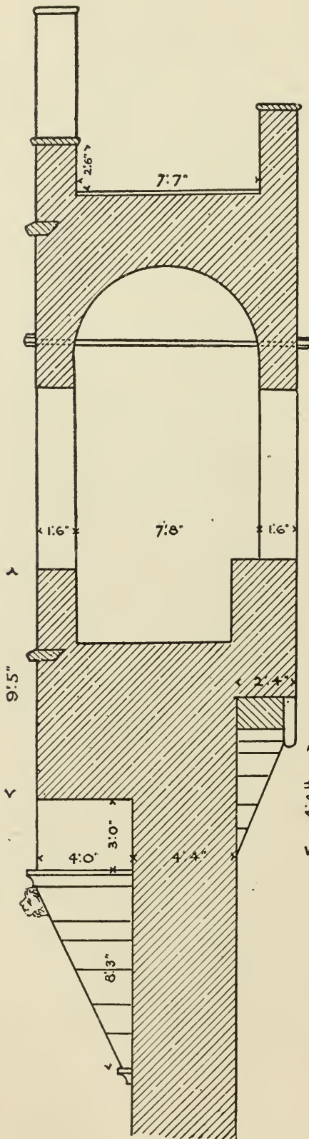
Fig. 432. Section of Main Cornice of Palazzo Vecchio.
