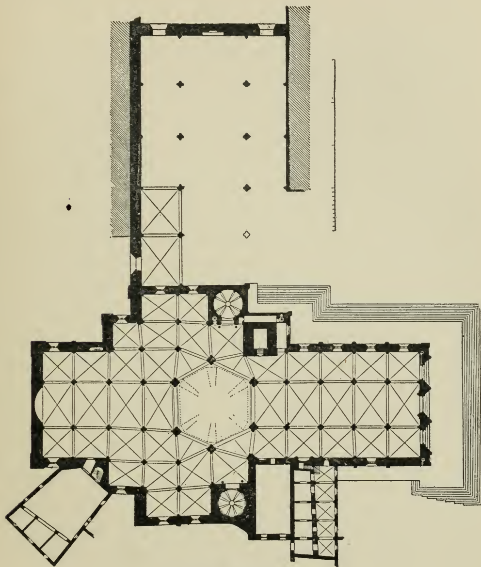
Fig. 353. Siena Cathedral.
