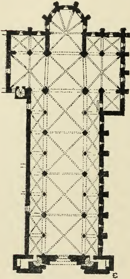
Fig. 338. Plan of S. Martino.
