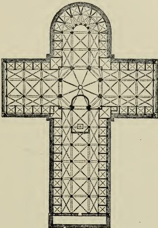
Fig. 377. Bologna. Original Plan of S. Petronio.
