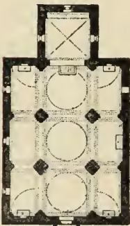
Fig. 251. Immaculati. Trani.
