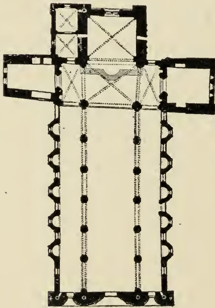
Fig. 358. Orvieto. Cathedral.
