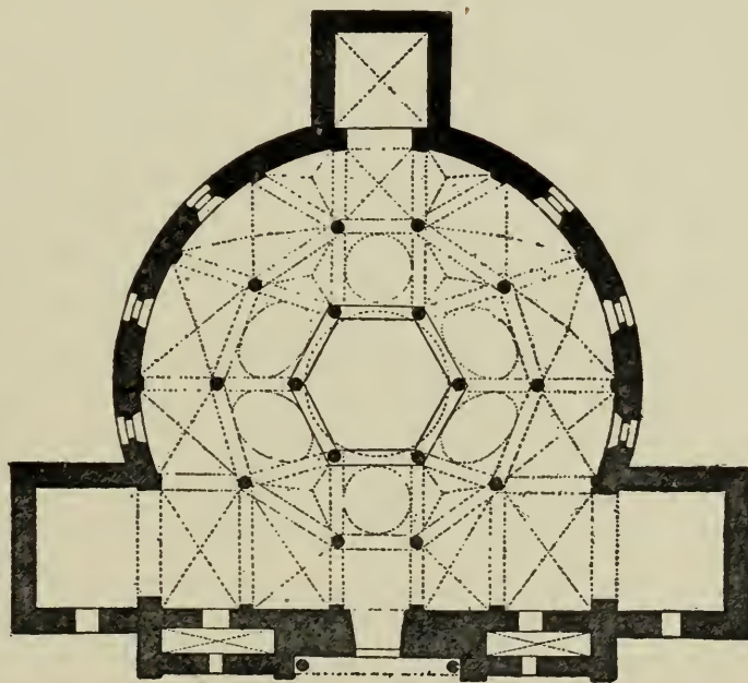
Fig. 258. Benevento. S. Sofia.
