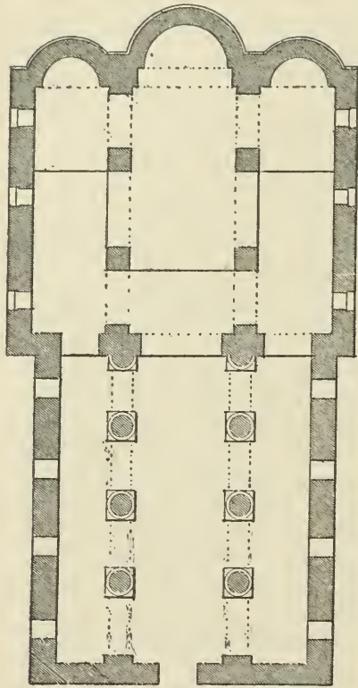
Fig. 308. Palermo. Chiesa dei Vespri.
