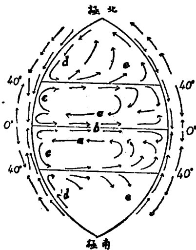
海流發達圖 (a) 赤道流 (b) 暖流 (c) 深流 (d) 赤道反流 (e) 泉流
