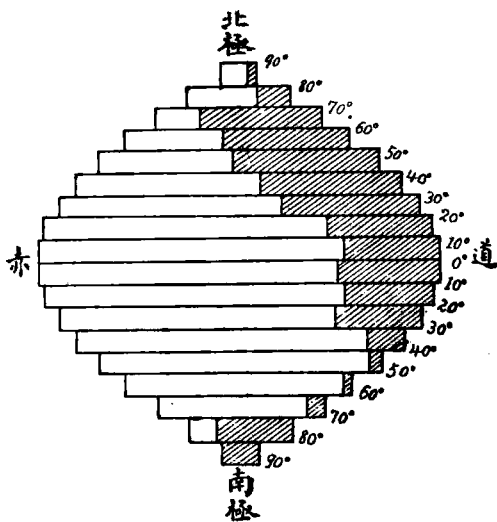
(面海部線無地陸部線有) 例比之積面陸海
