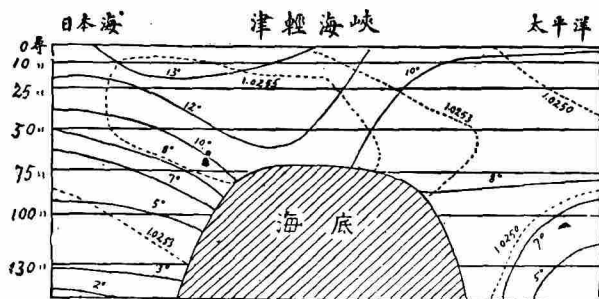
滋青兩側水溫之變化
