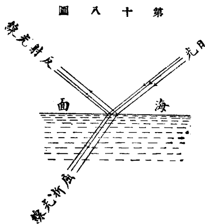
日光射與光線折屈線光射投
