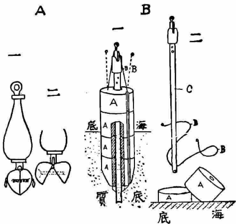
底質探取器
