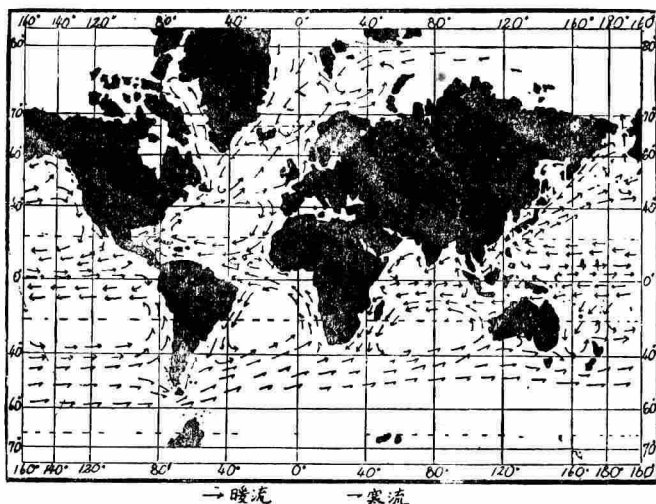
三 大 洋 之 海 流
