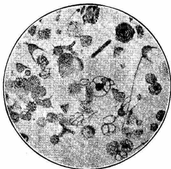
放射蟲沈源
