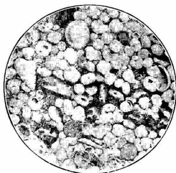
有孔蟲沈澱
