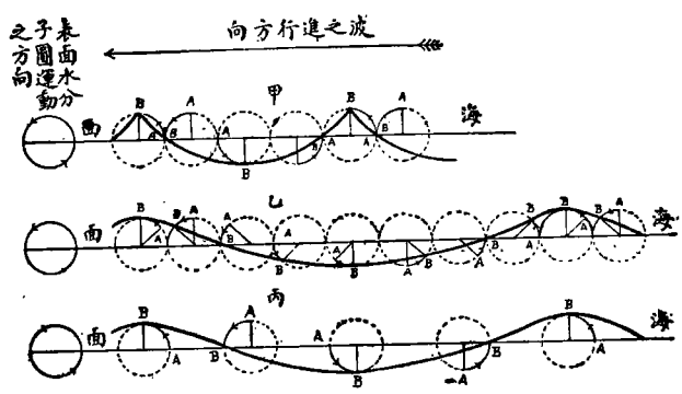
波浪之周期、波長、速度之關係圖
