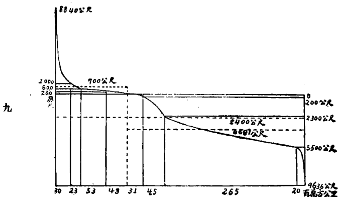
海 陸 高 低 圖
