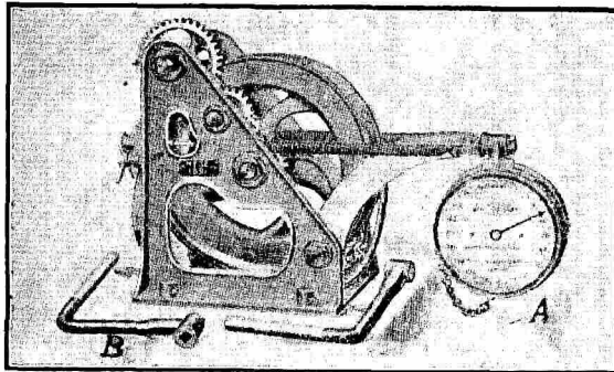
卡爾斯測深器 (A) 測深表 (B) 柄搖
