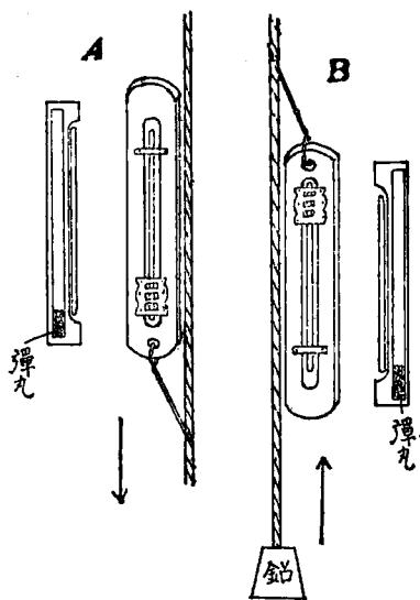
倒轉寒暖計 (A) 中下沈 (B) 中引出
